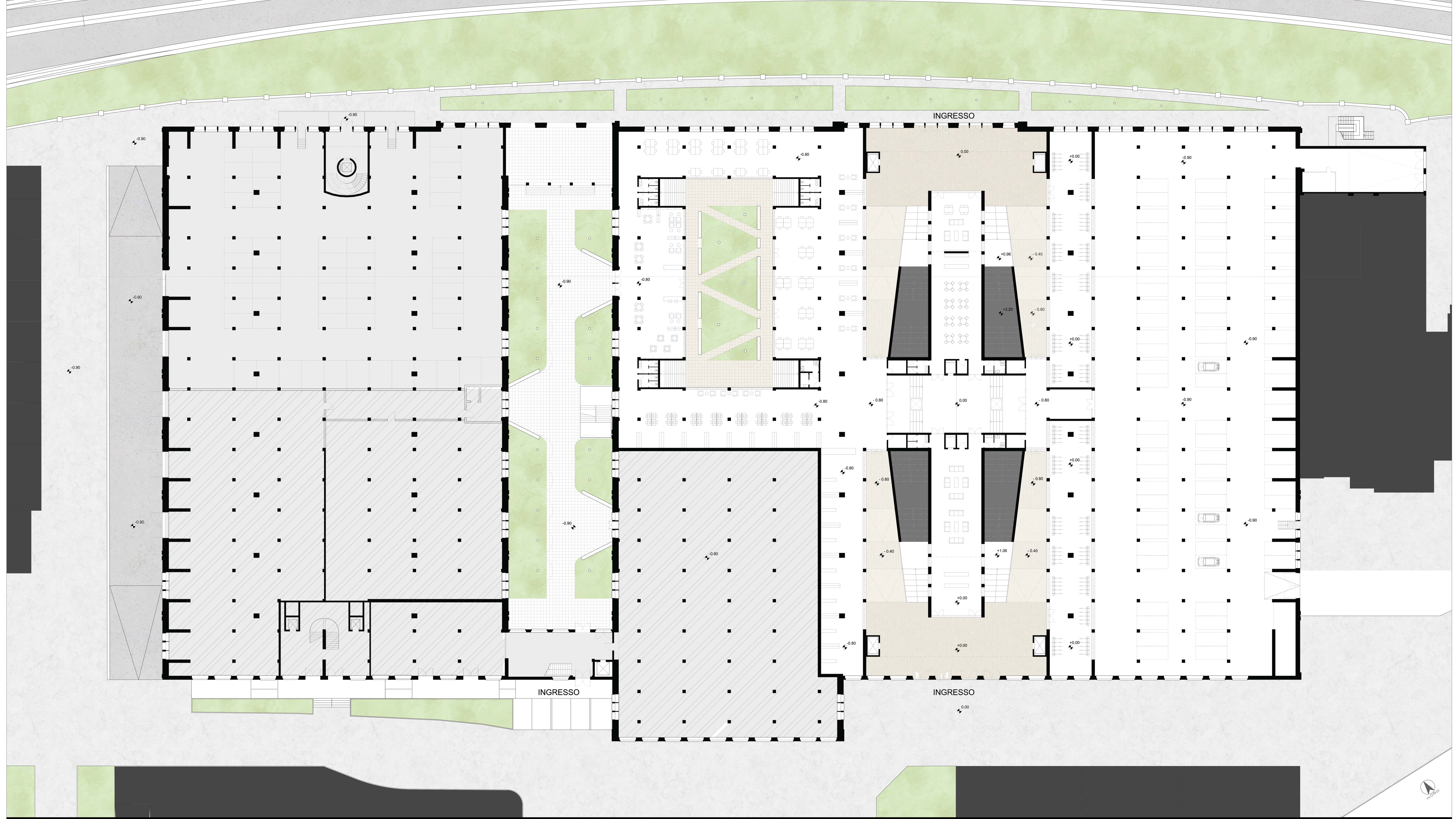
PIANTA PIANO INTERRATO SCALA 1:200
