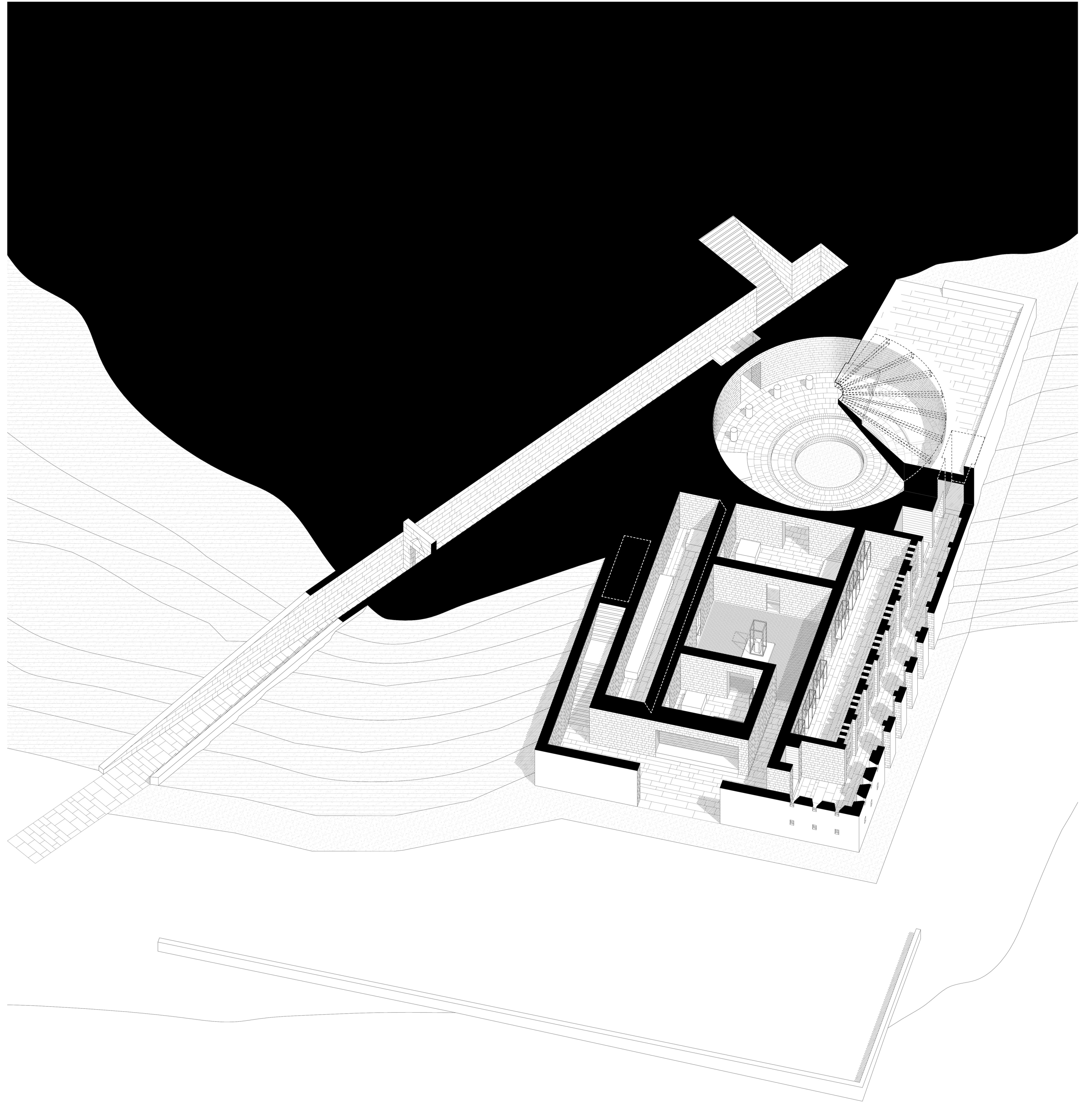
SPACCATO ASSONOMETRICO SPAZIO MUSEALE
