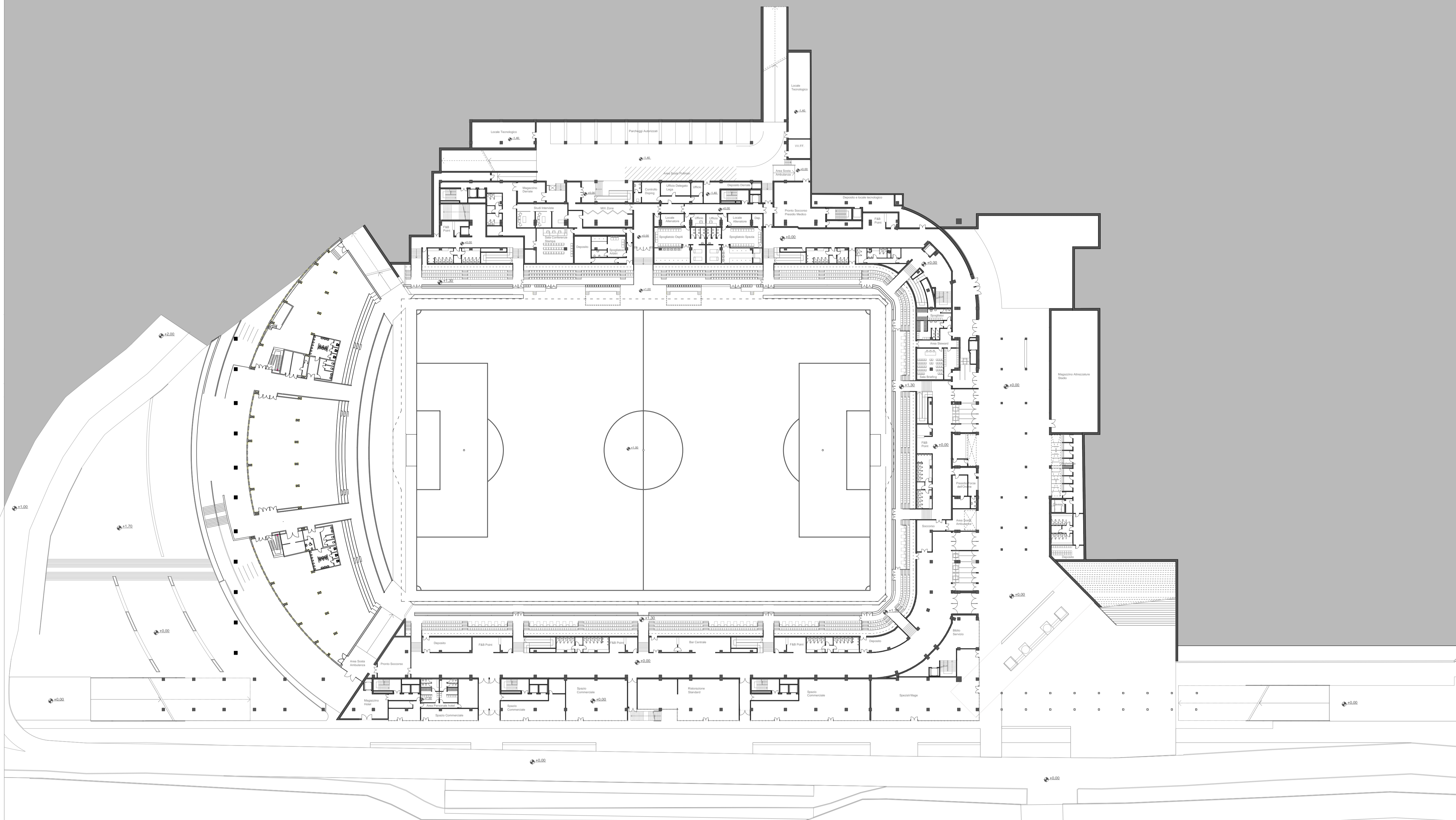
PIANTA PIANO TERRA Scala 1:500
