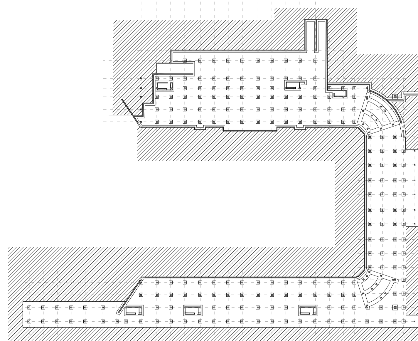
SCHEMA STRUTTURALE
