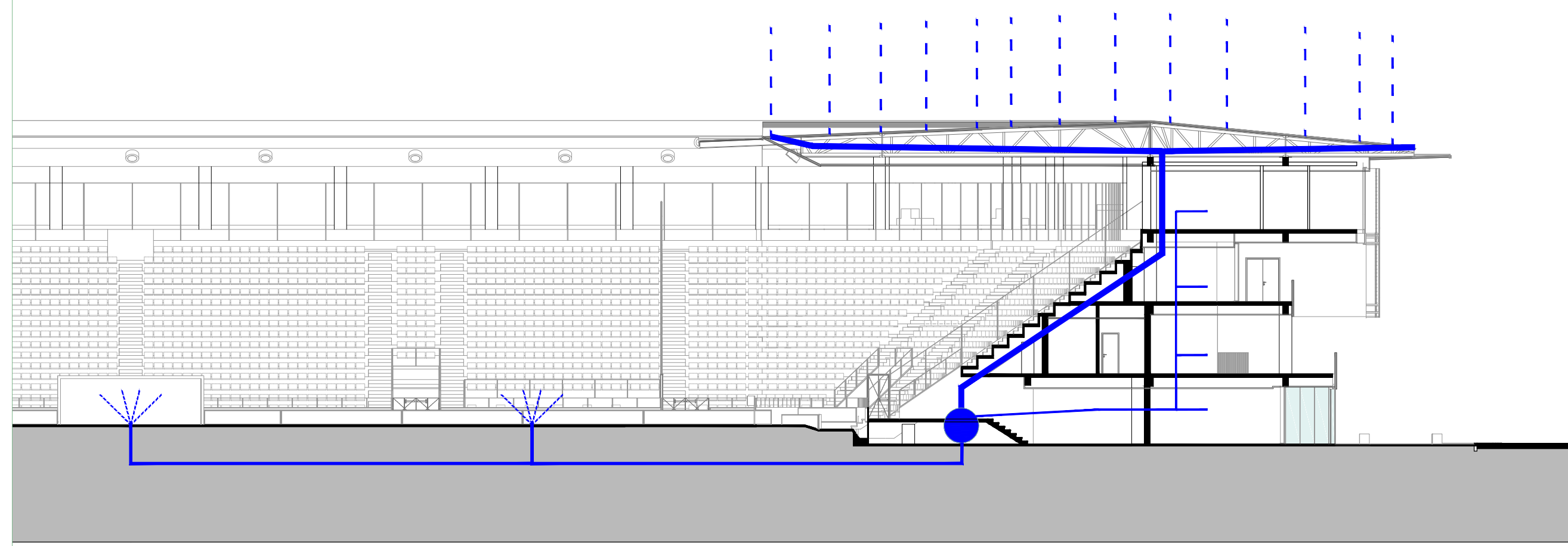
SCHEMA RACCOLTA E RIUSO ACQUE PIOVANE
