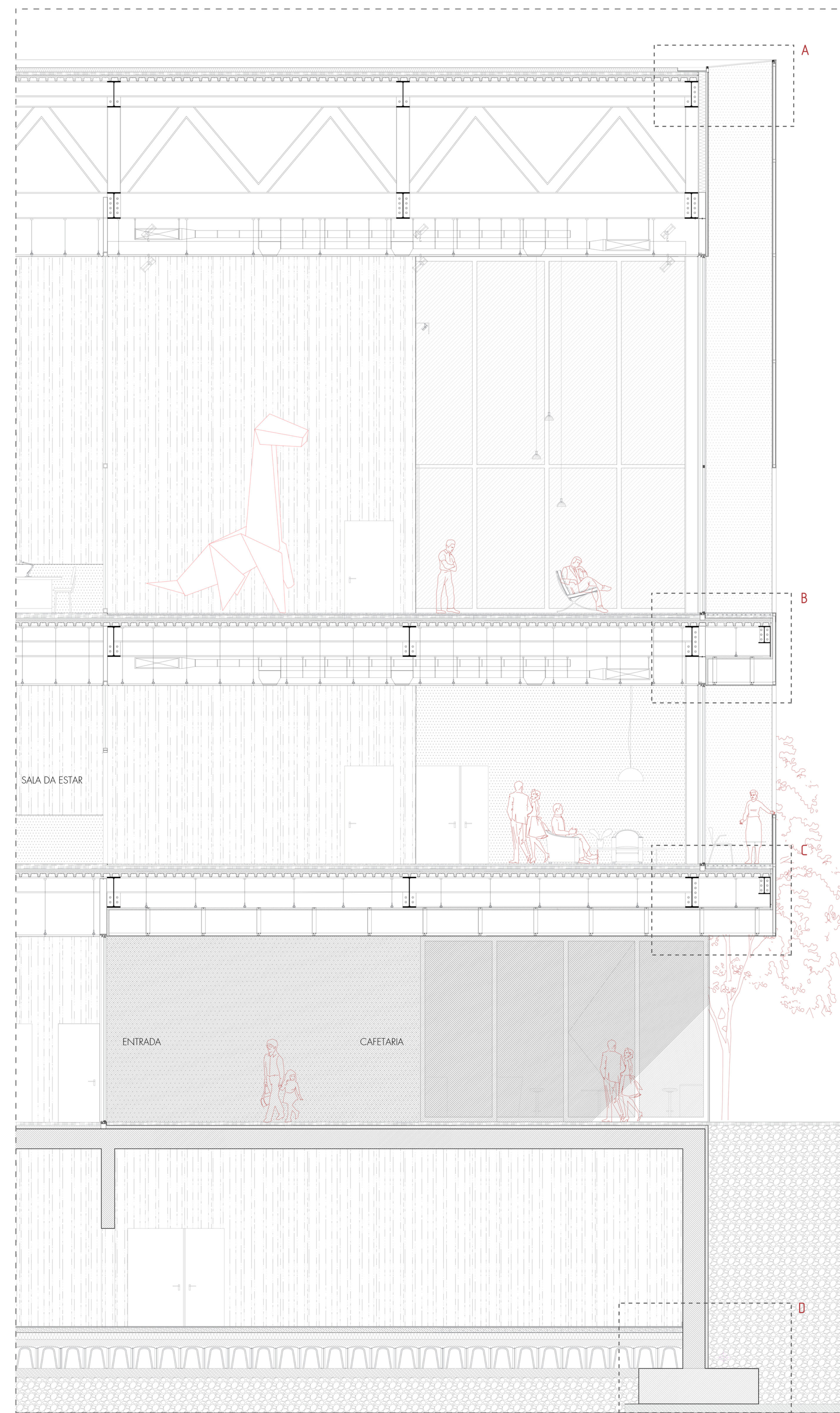
SEZIONE AA'
