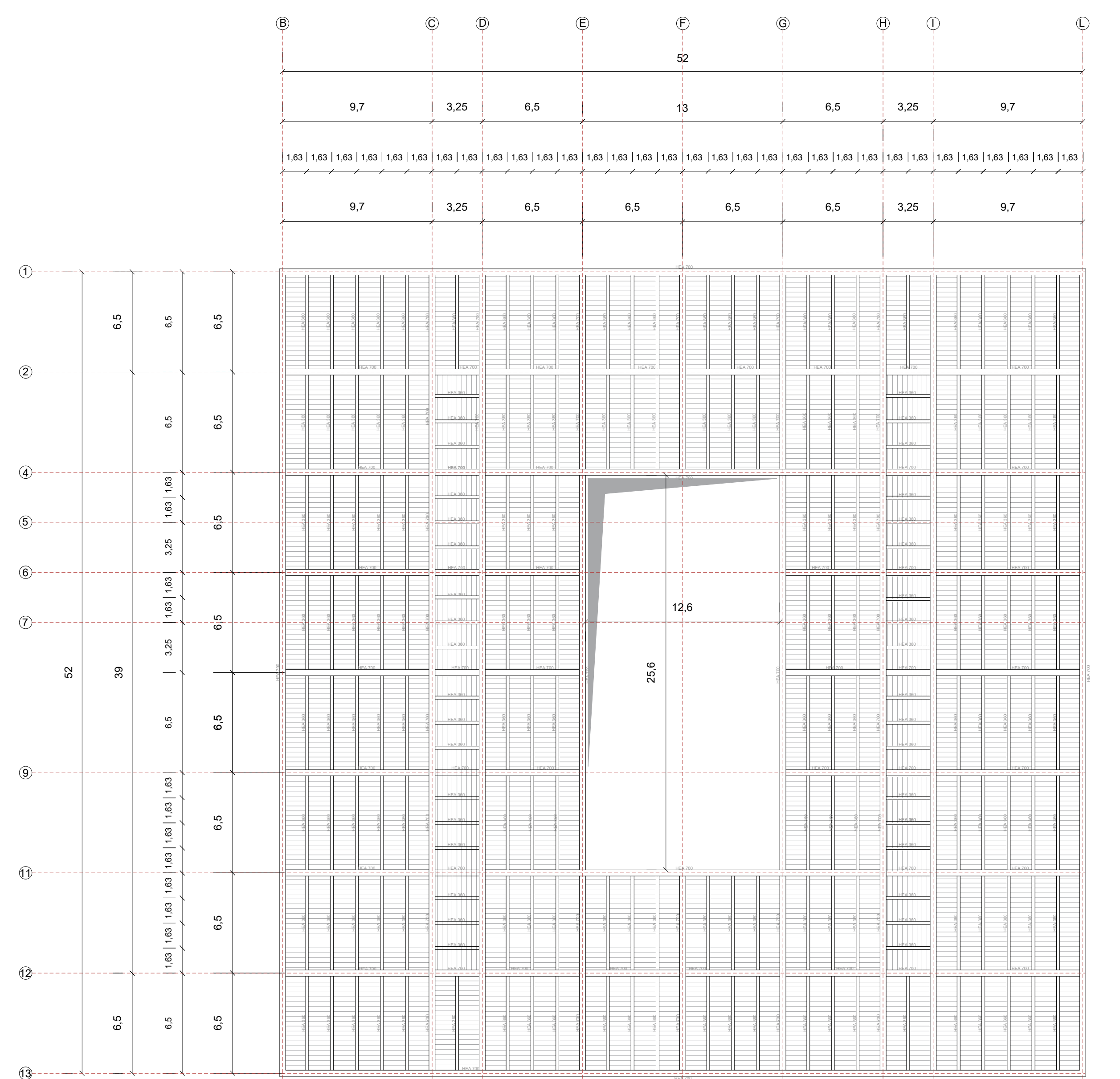
COPERTURA GRATICCIO RETICOLARE +24,50m
