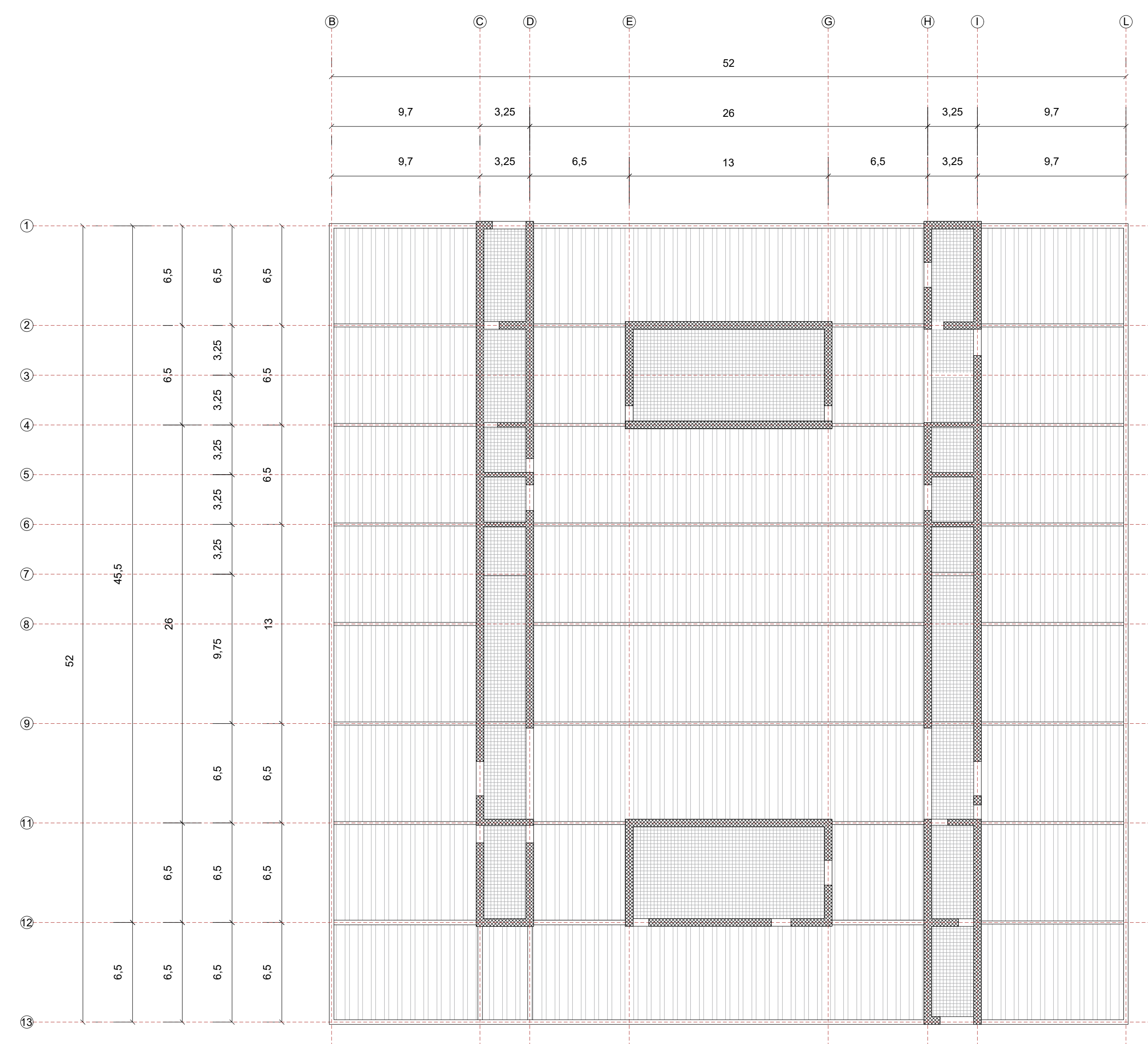
PIANO TERRA +0,00m
