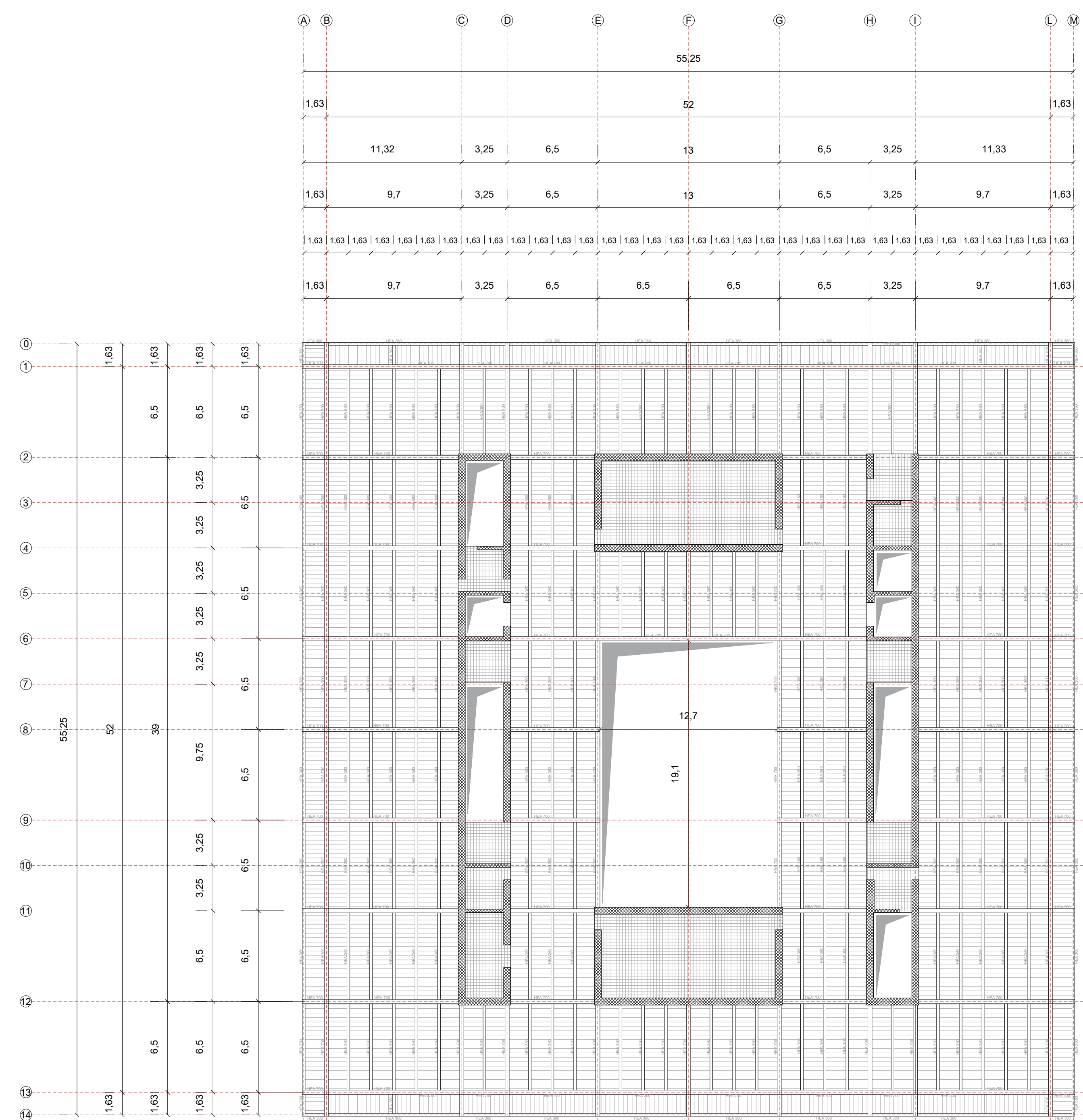
PIANO PRIMO +5,50m
