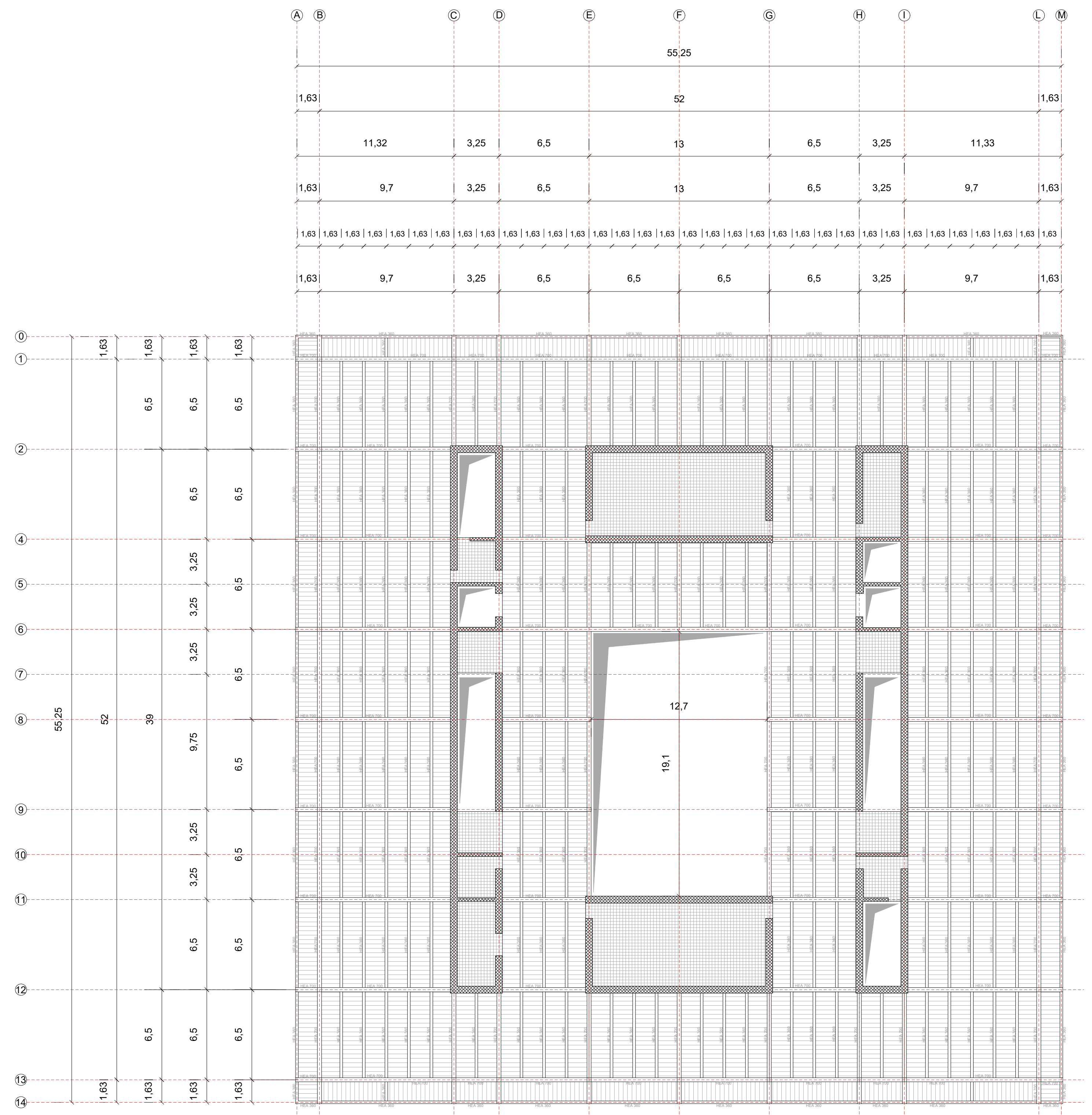
PIANO SECONDO +11,00m
