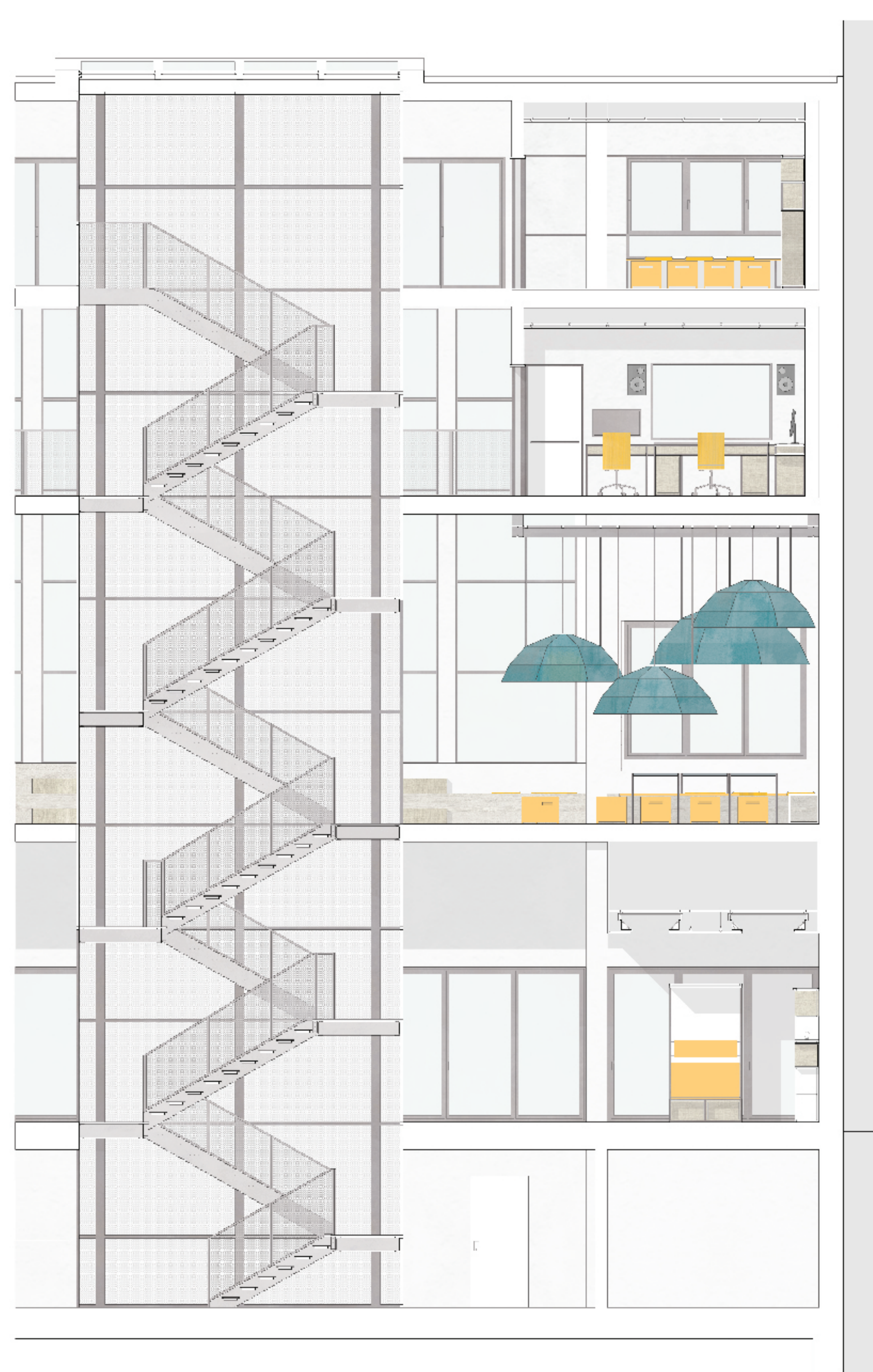
SEZIONE B-B
