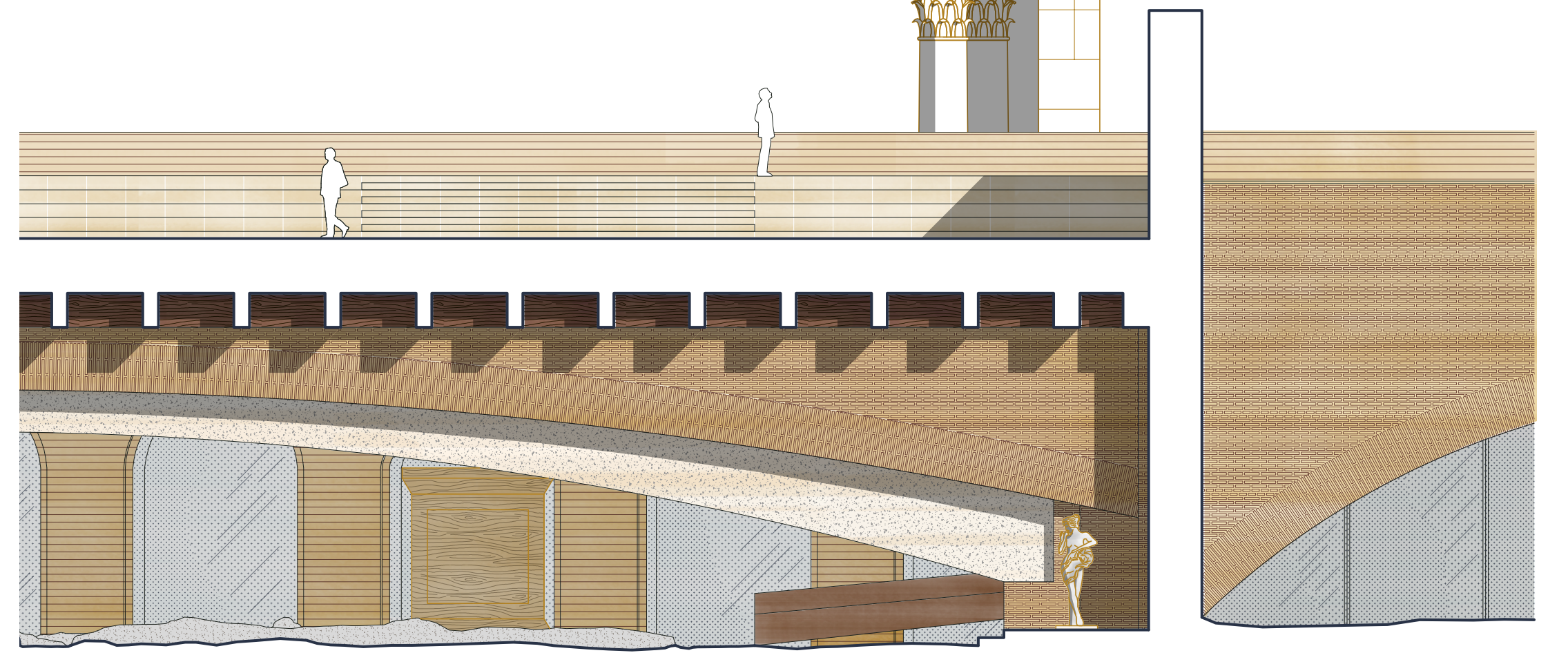
immagine X, XI, XII, XIII. RIDEFINIZIONE DEI LIMITI - pianta e sezione trasversale, scala 1:100
