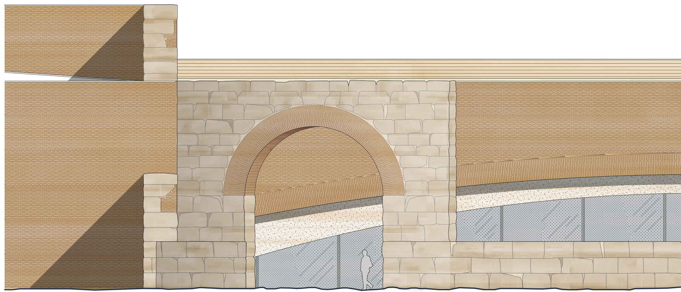
immagine X, XI, XII, XIII. RIDEFINIZIONE DEI LIMITI - pianta e sezione trasversale, scala 1:100
