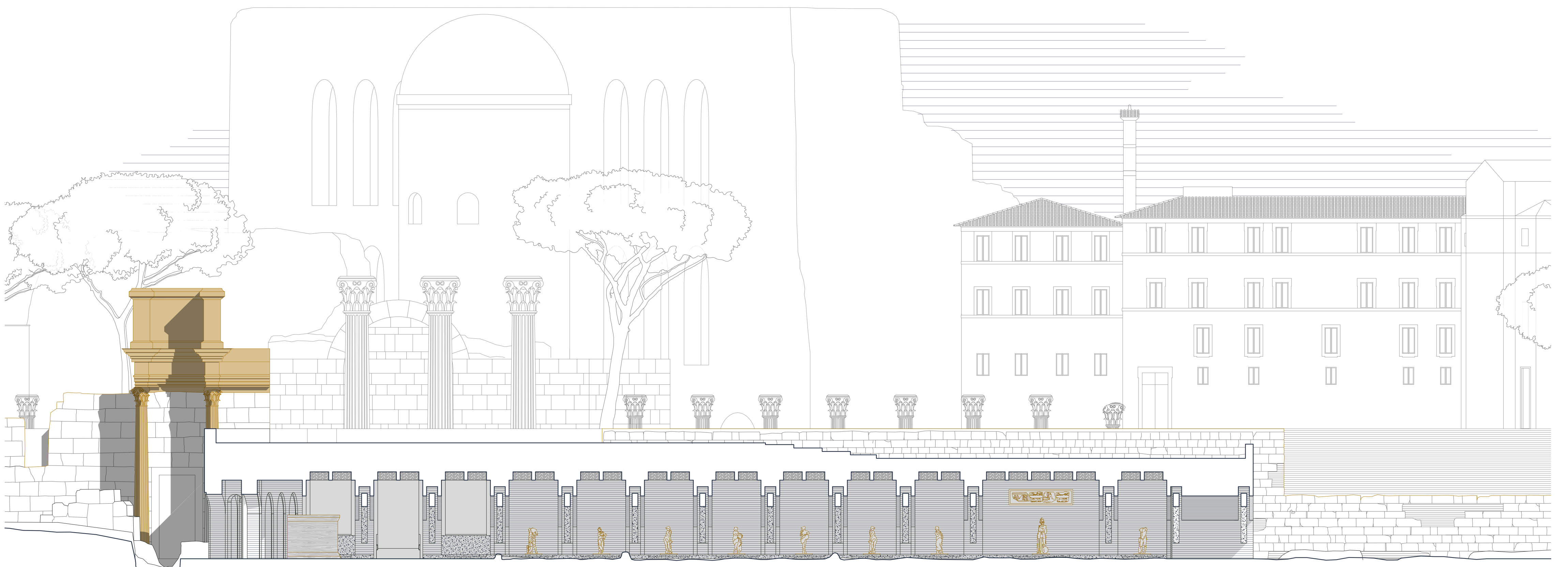
immagine XV. RIDEFINIZIONE DELLA CONTINUITÀ SPAZIALE - sezione longitudinale, scala 1:200
