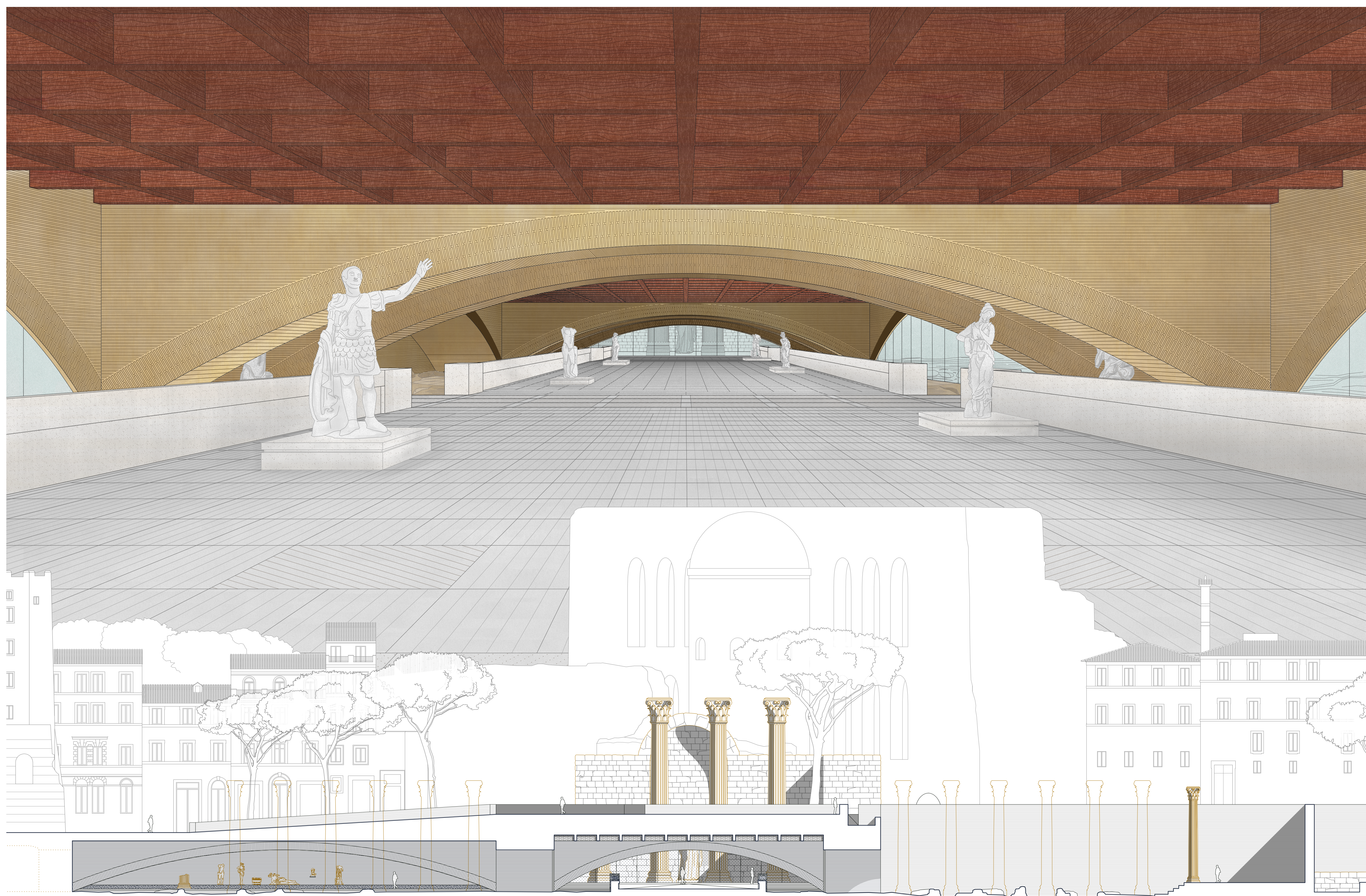
immagine XVI, XVII. RIDEFINIZIONE DELLA SIMMETRIA SPAZIALE - vista e sezione trasversale, scala 1:250
