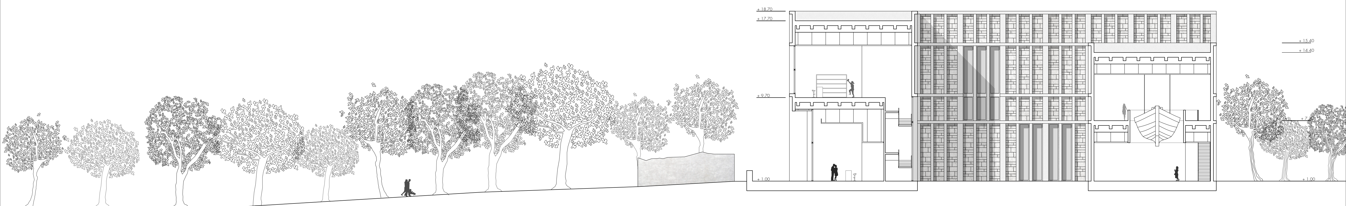
SEZIONE HH'
