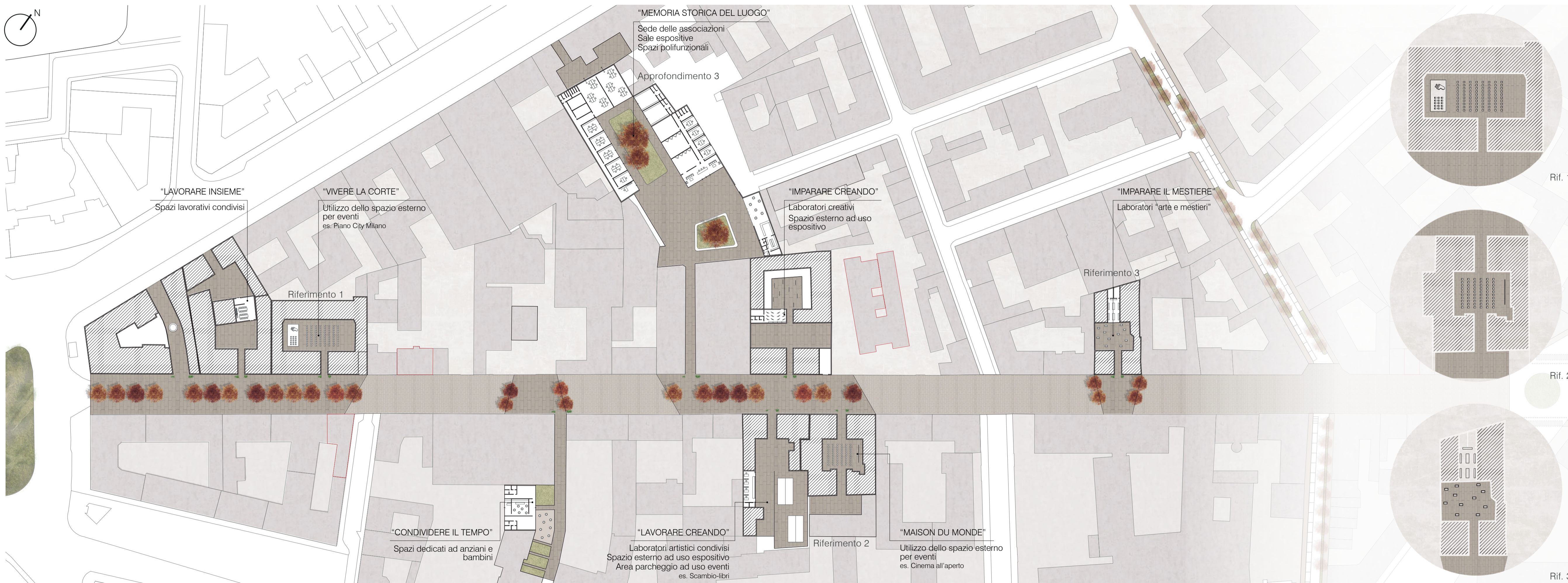
Pianta primo tratto Via Padova - Scala 1:1000
