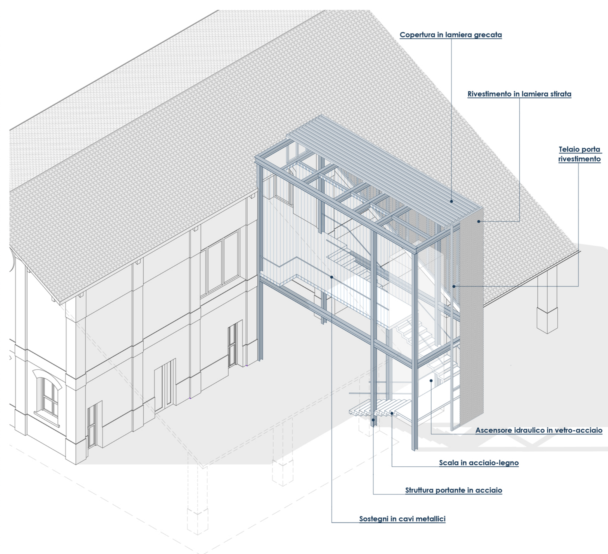
Schema strutturale scala
