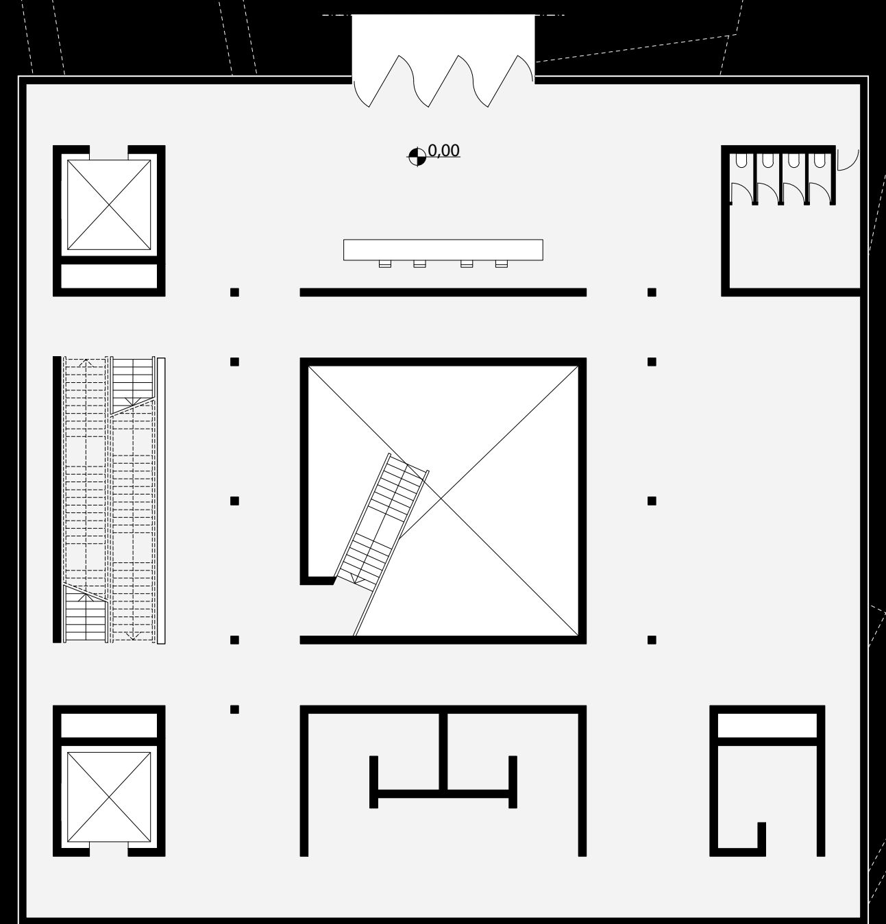
ATTACCO A TERRA CUBO STEREOTOMICO
