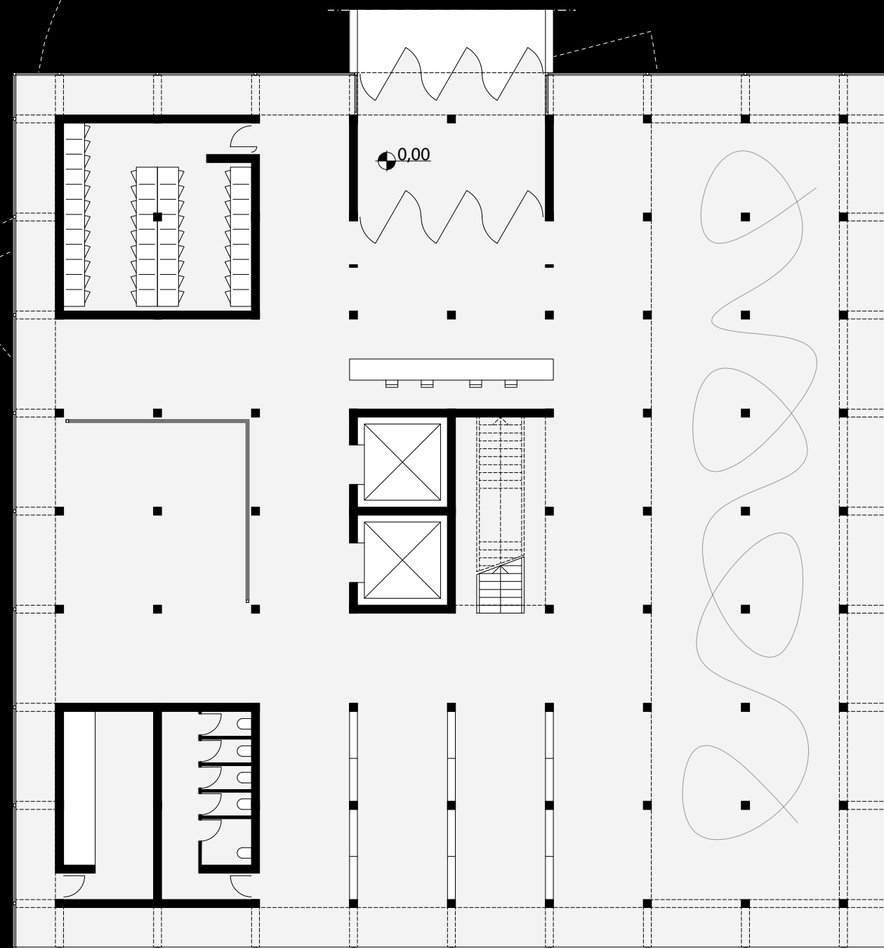
ATTACCO A TERRA CUBO TETTONICO
