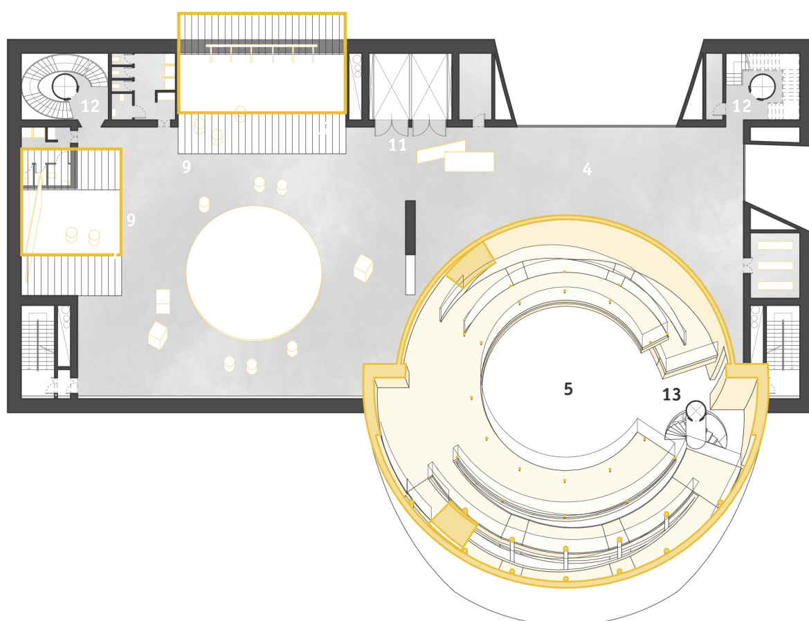
Pianta a quota +36m piano sale prova
