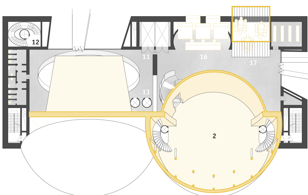
Pianta a quota +31,5m piano palco
