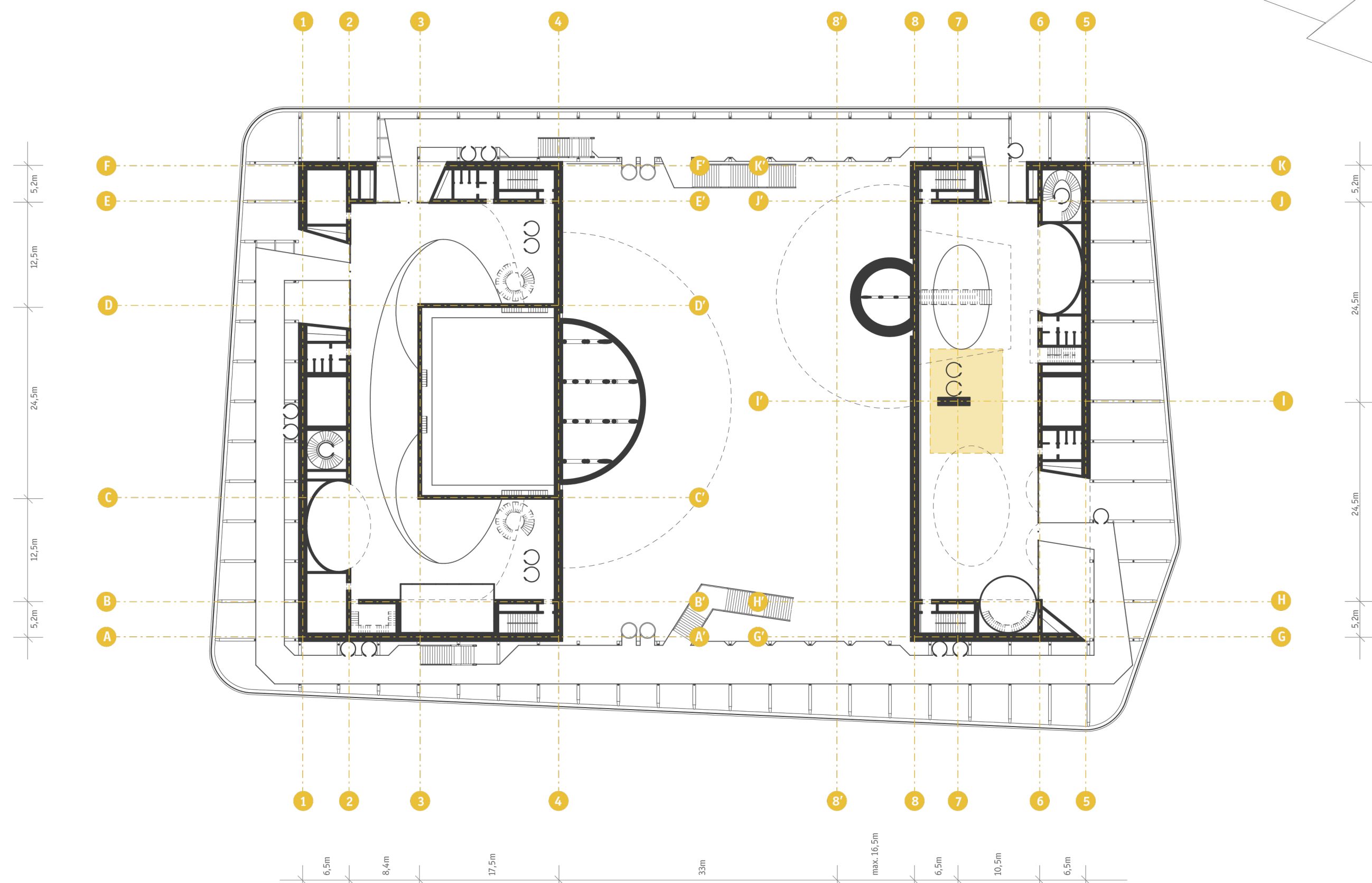
Pianta fili-picchetti (a quota +4,5m) scala 1:500
