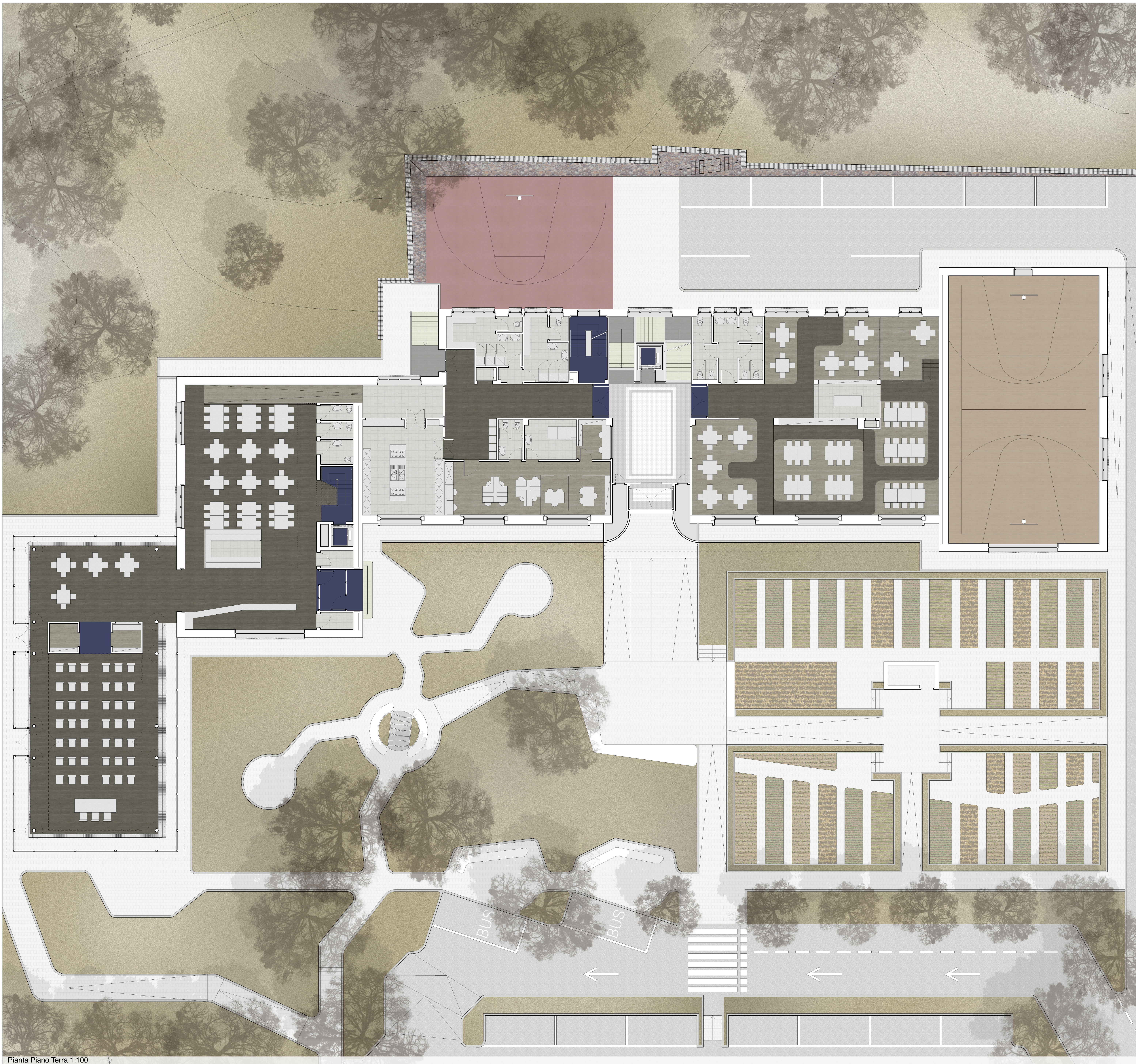
Pianta Piano Terra 1:100
