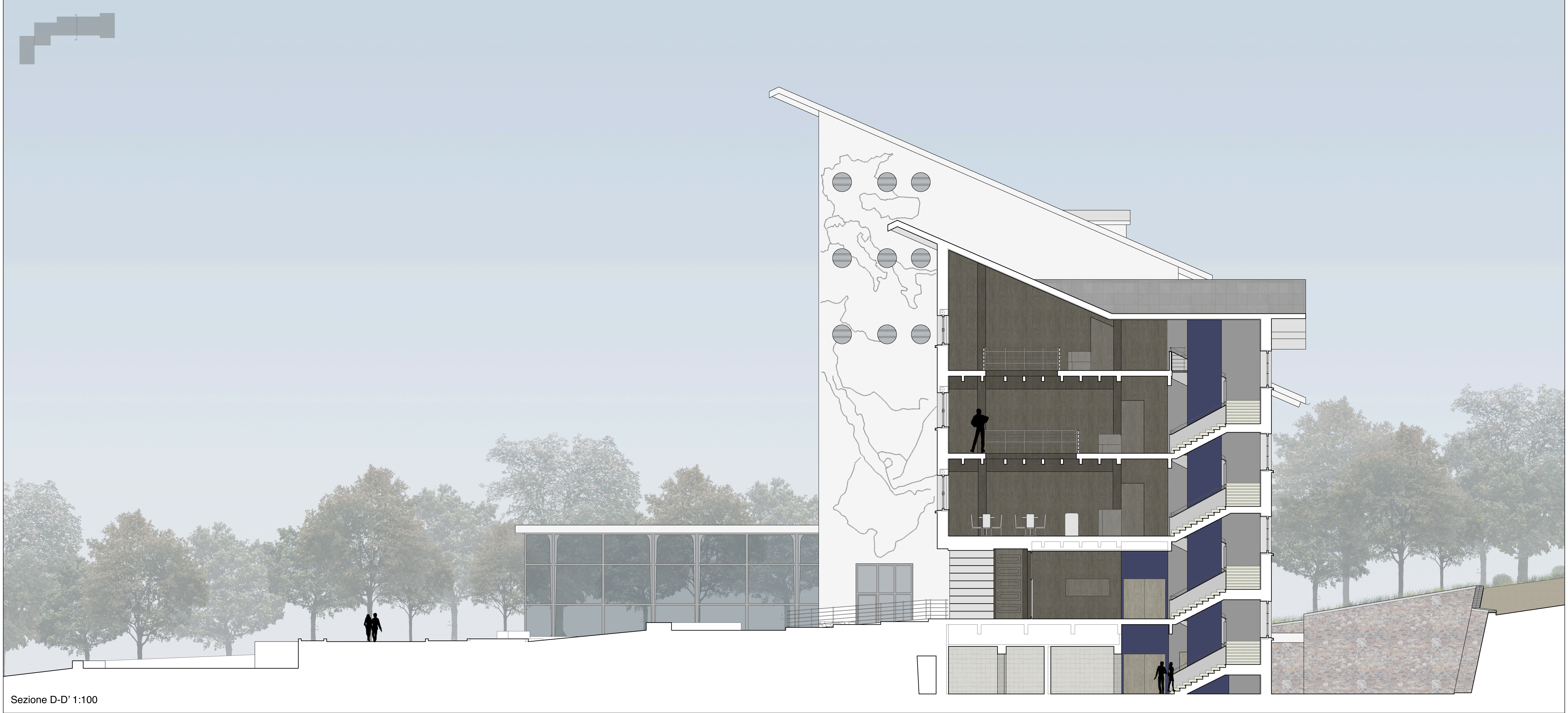
Sezione D-D' 1:100
