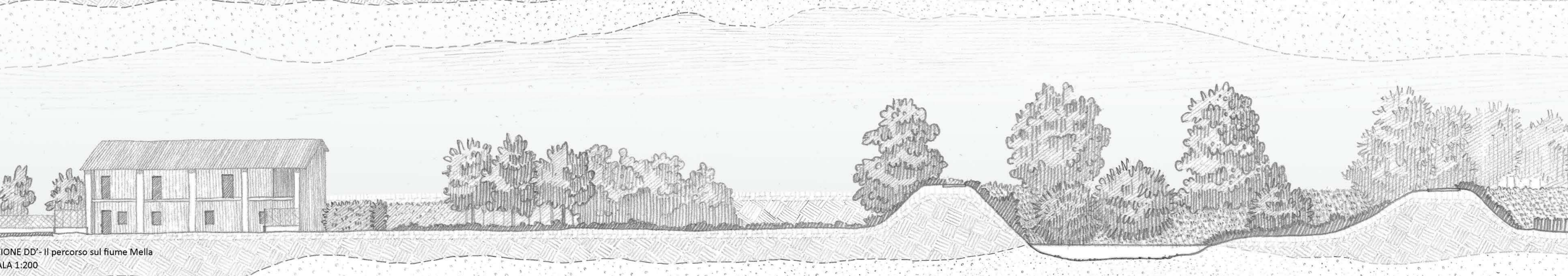
SEZIONE CC' - Percorso lungo il fontanile Biscia SCALA 1:200
