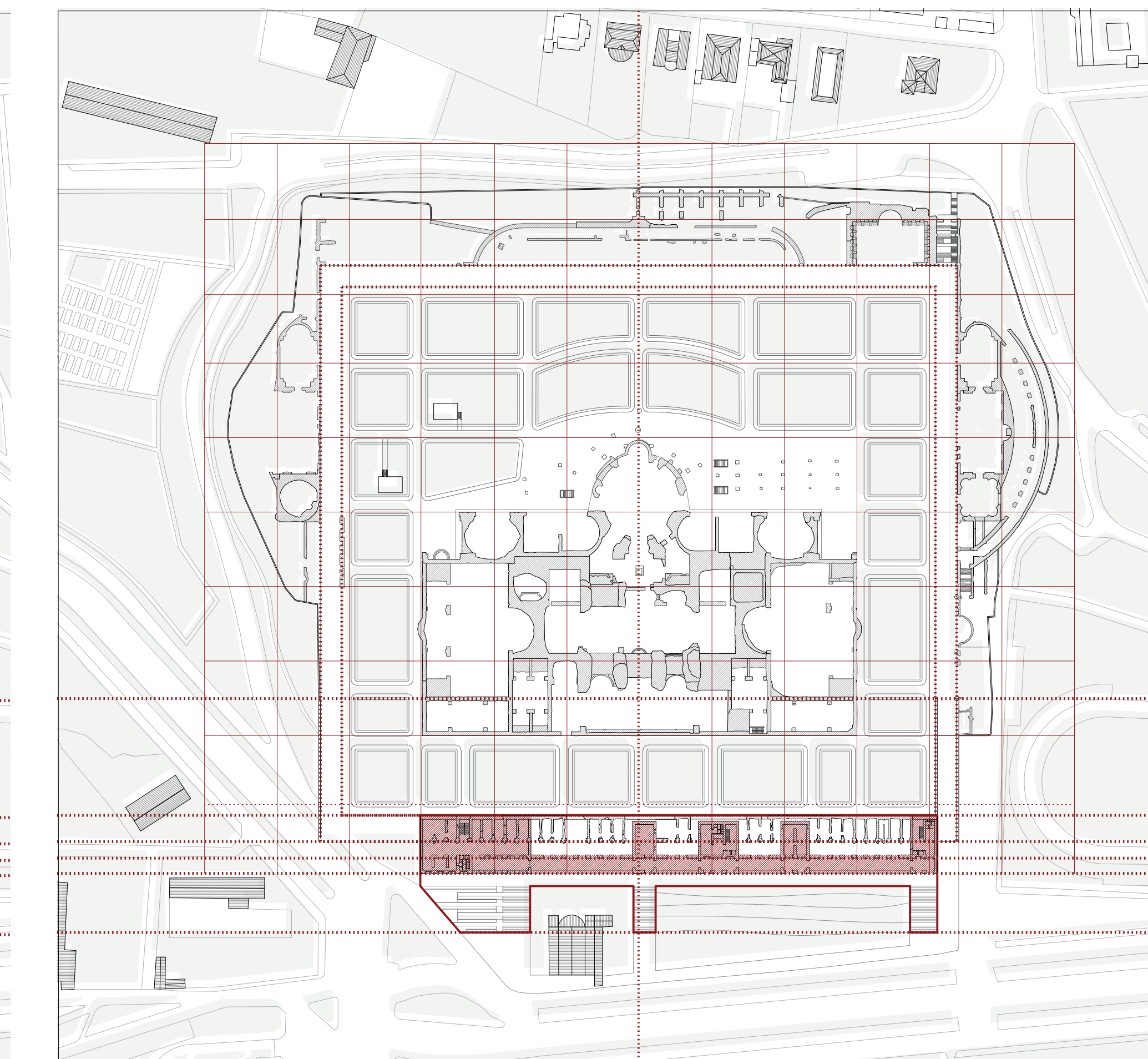
Terme di Caracalla - stato di progetto Pianta quota scavo archeologico delle tabernae scala 1:2000
