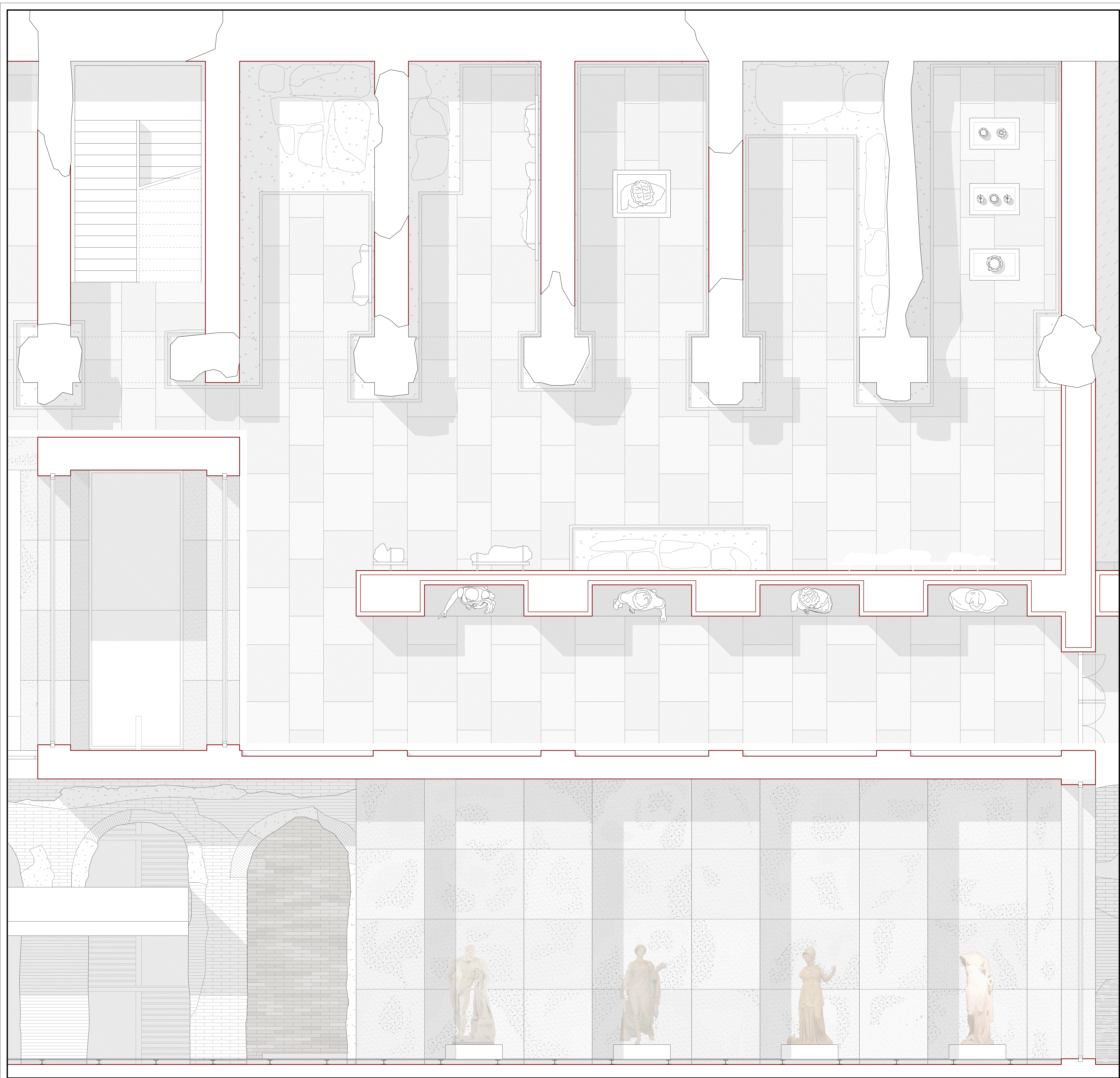
PIANTA E SEZIONE DEL MUSEO scala 1:50
