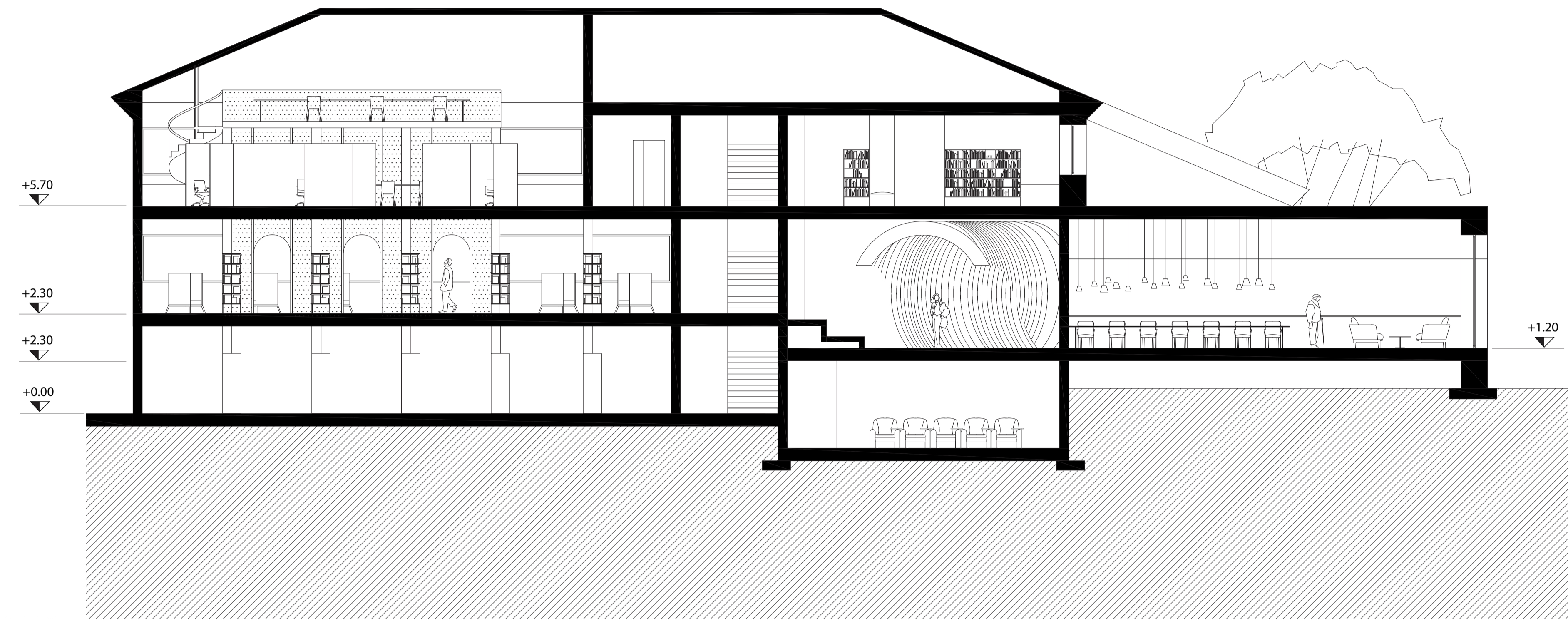
SEZIONE AA'
