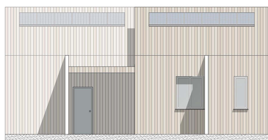
PROSPETTO SUD Scala 1:100
