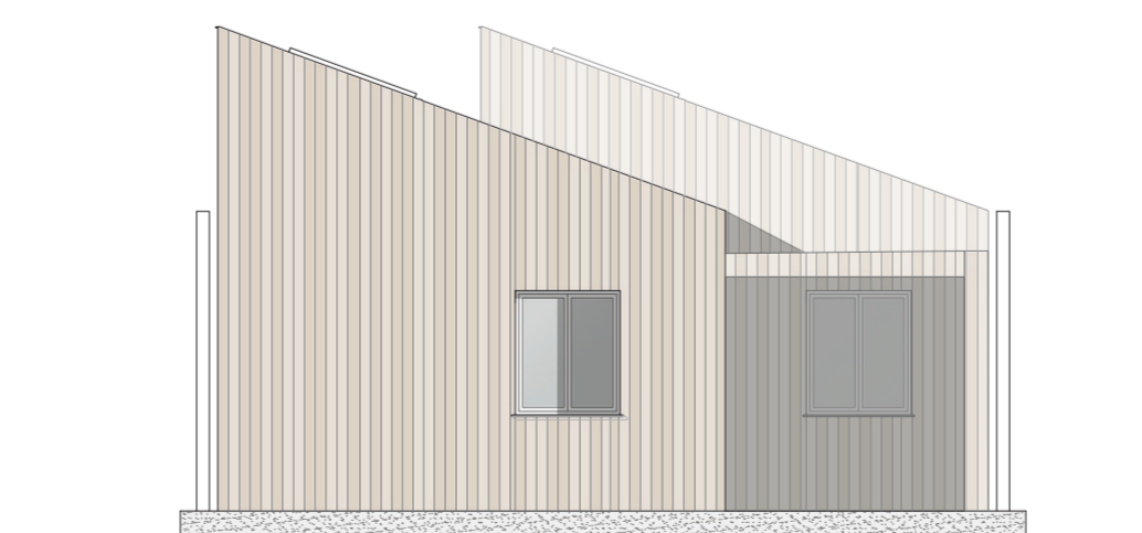
PROSPETTO OVEST Scala 1:100
