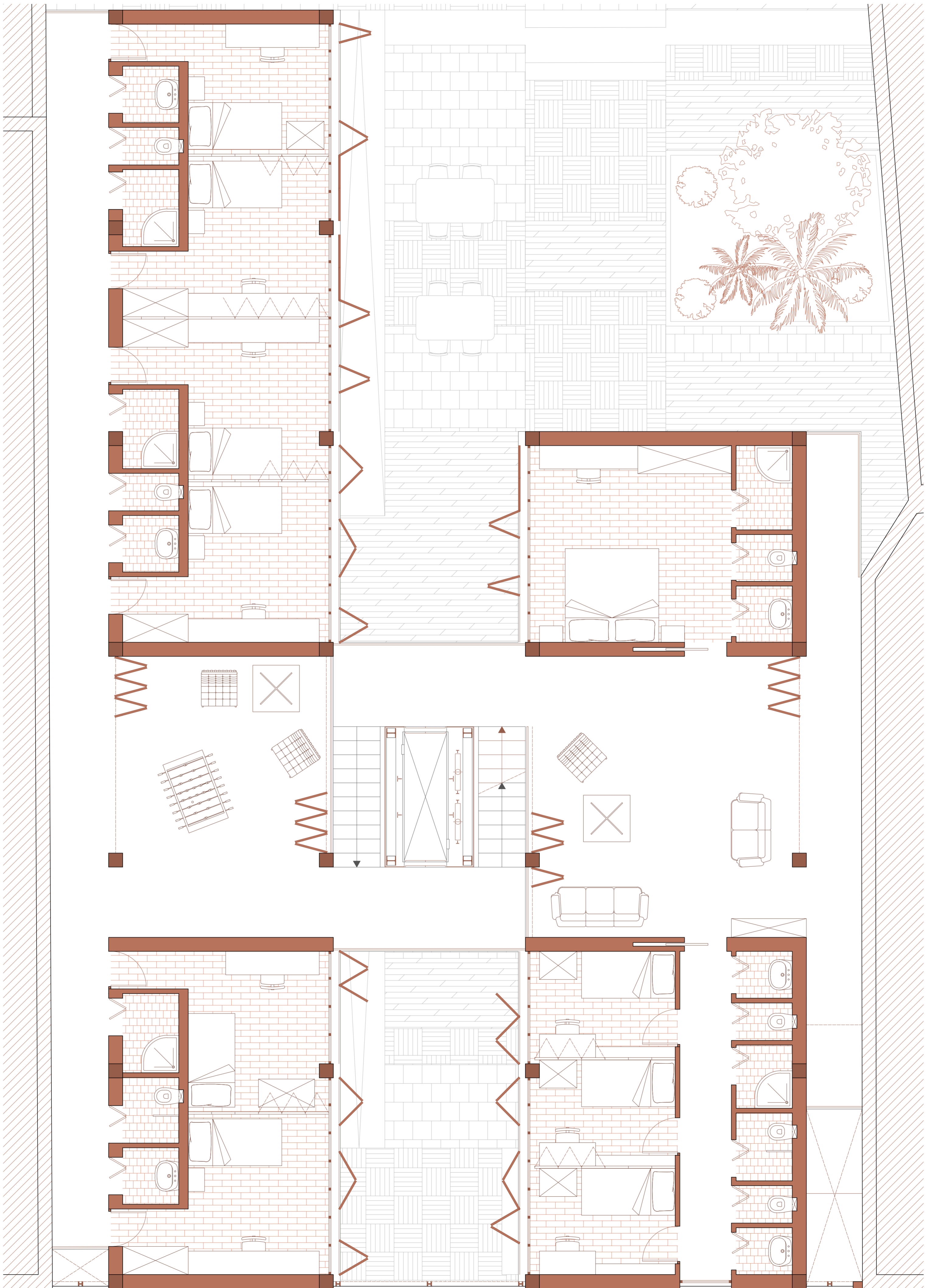
Pianta Primo Piano scala 1:50
