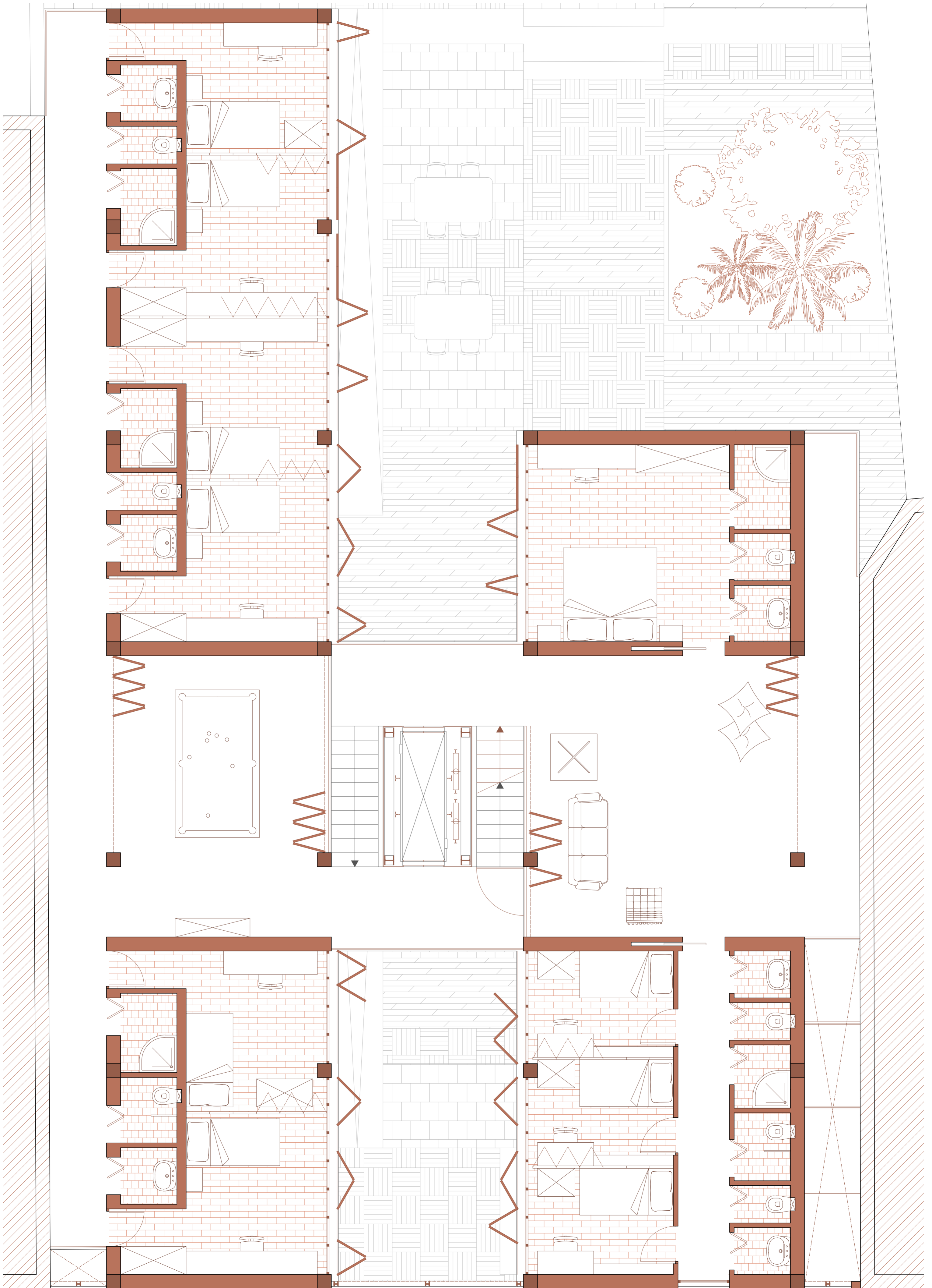
Pianta Terzo Piano scala 1:50
