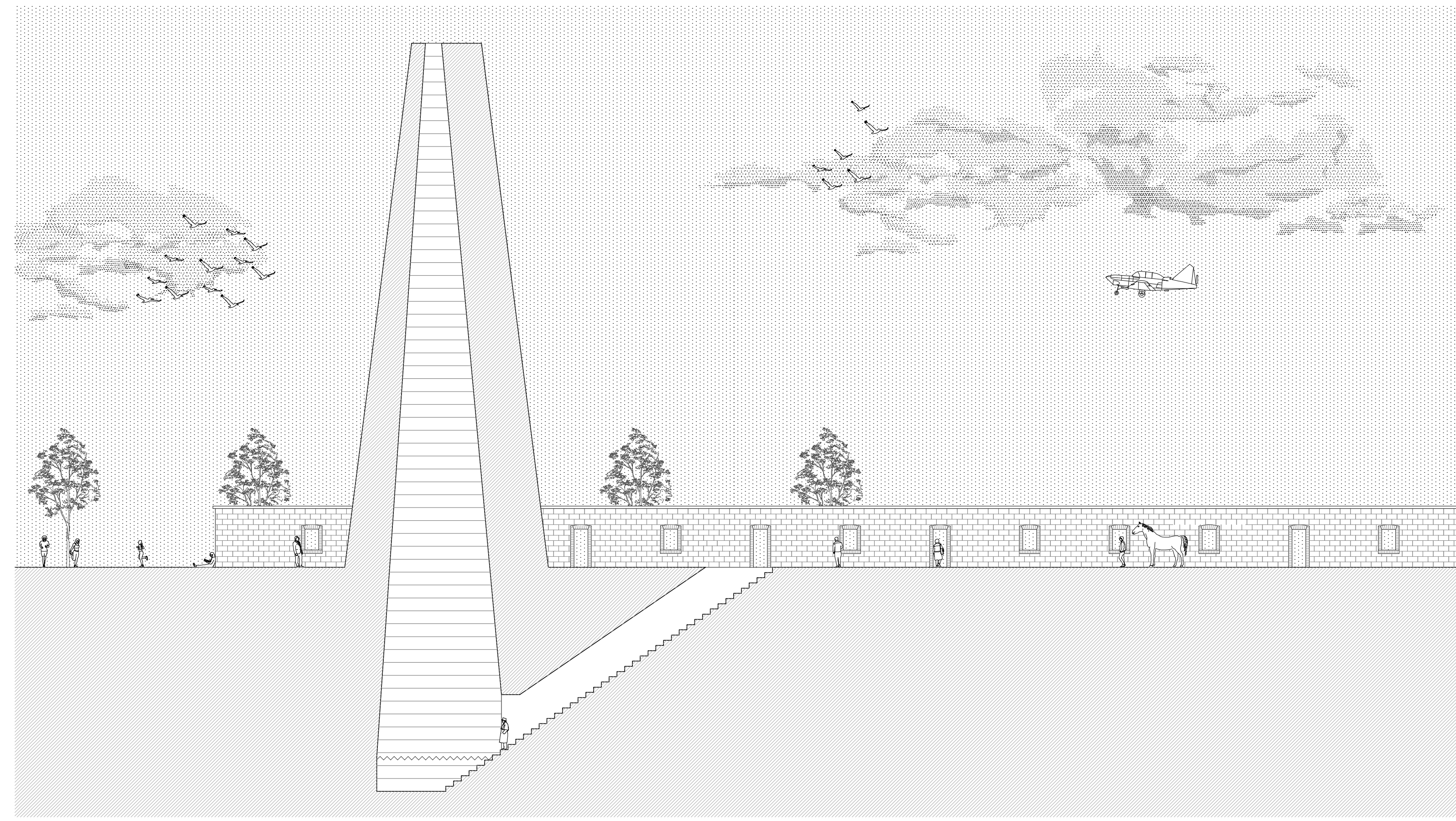
tavola XXI | batteria roccetta. lido di venezia progetto, pianta, sezione, scala 1:200; esploso assonometrico, assonometria
