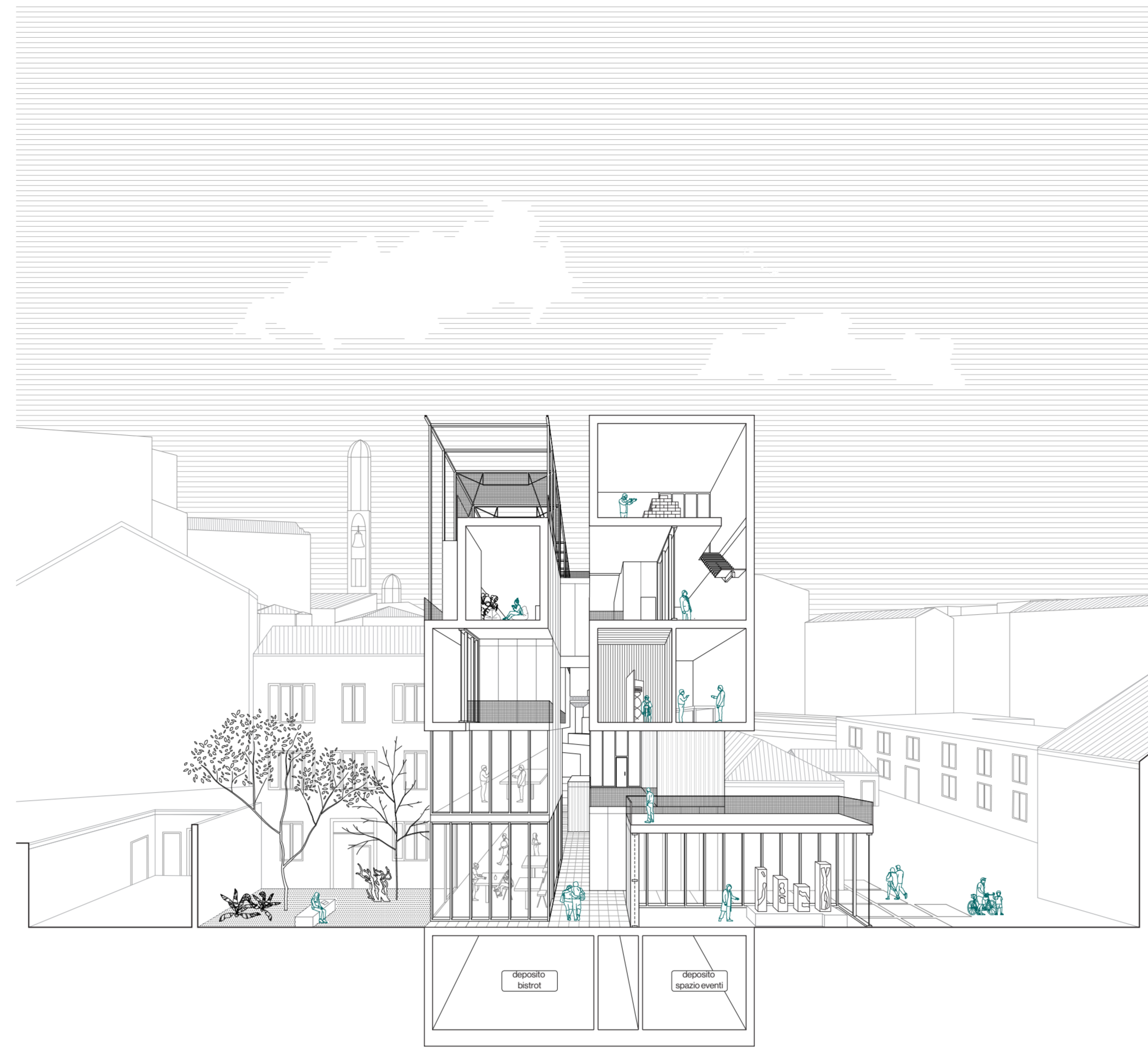
sezione F-F
