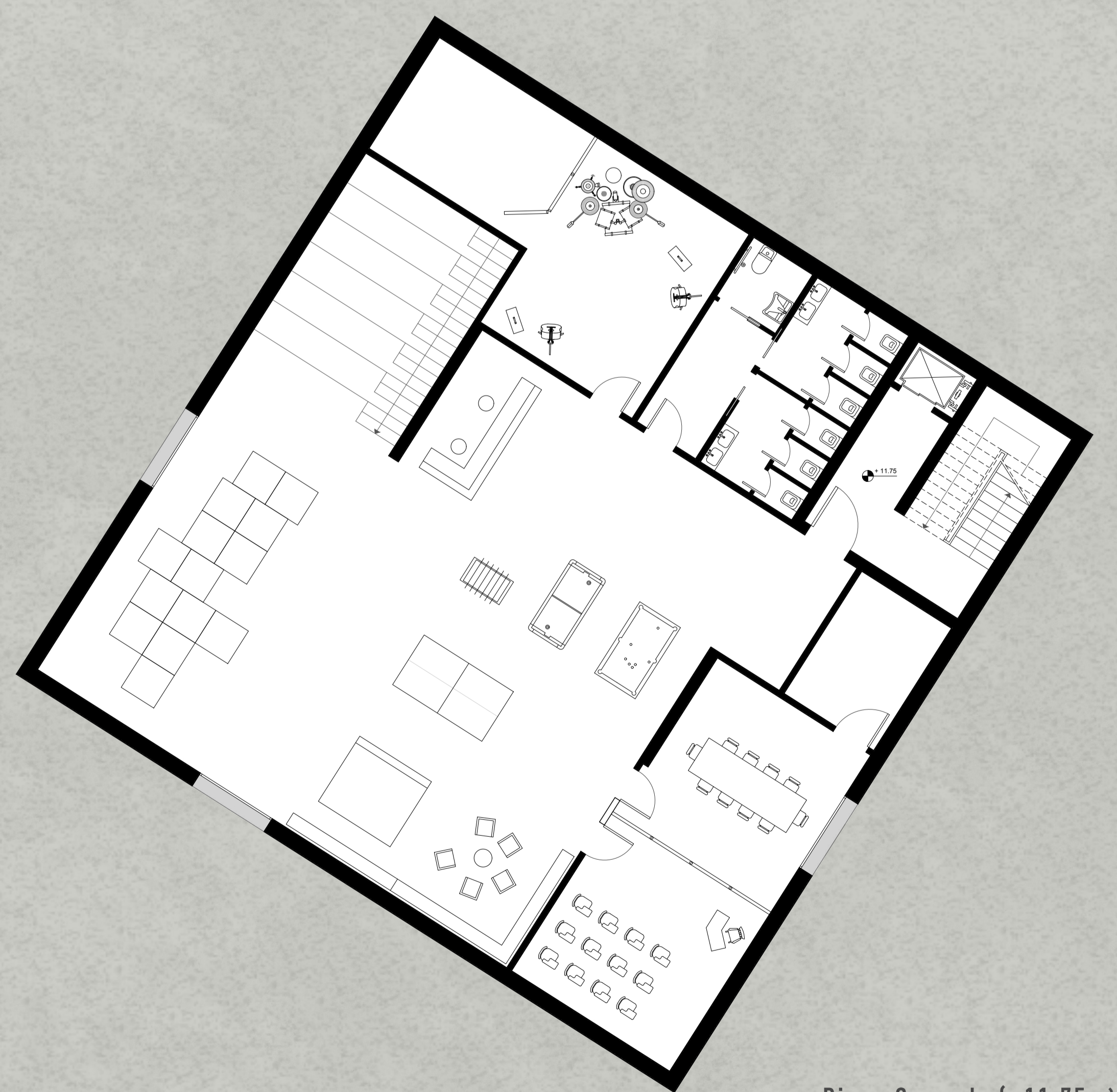
Piano Secondo (+11.75m) - spazi ricreativi comuni - sala prove - aule polifunzionali - magazzini
