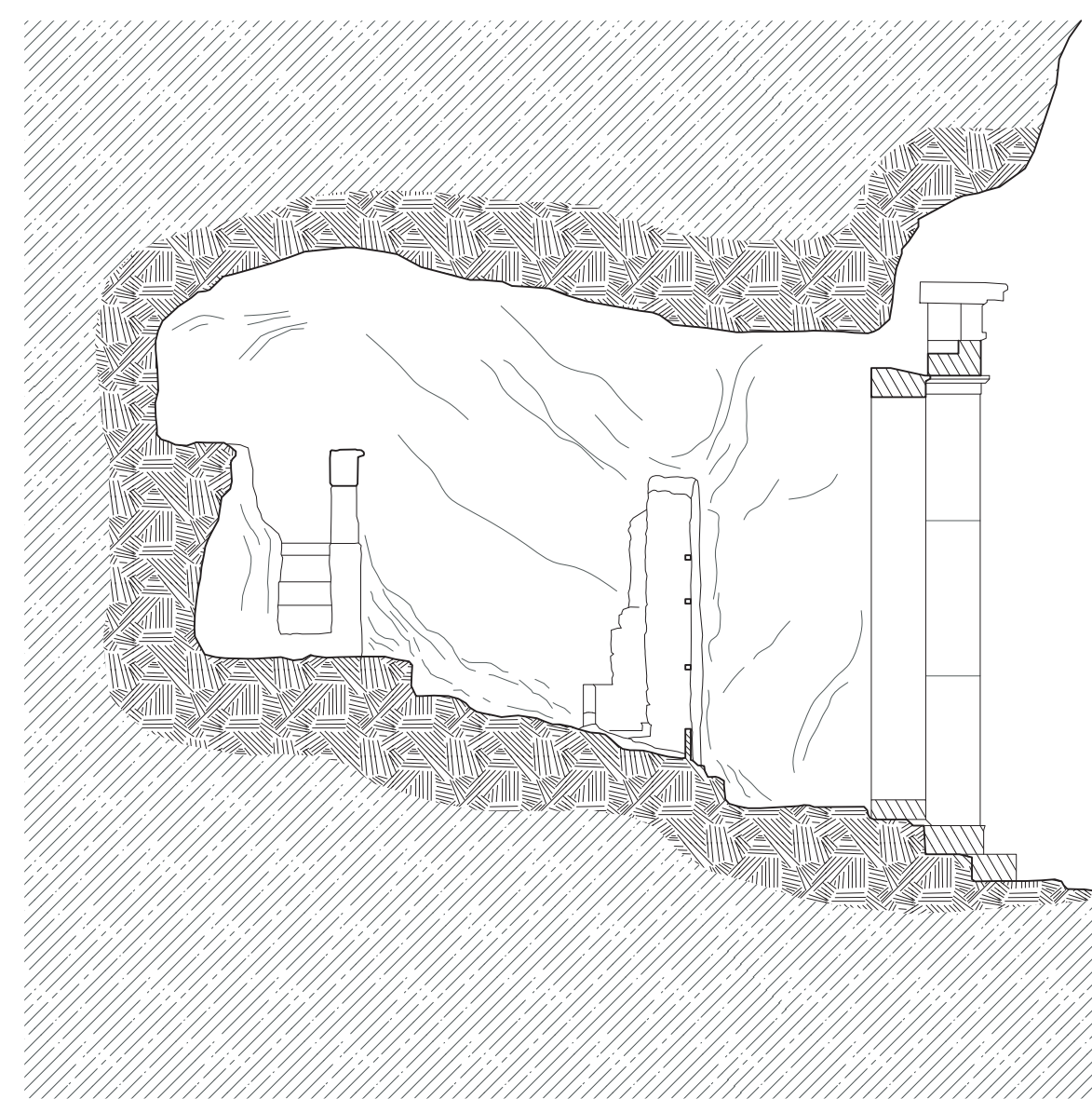
4 Monumento Coregio di Trasillo 320 - 319 a.C. pianta e sezione
