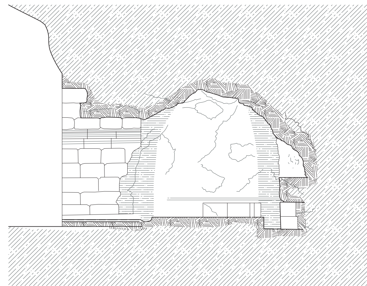
5 Fonte di Halirrhothios IV secolo a.C. pianta e sezione
