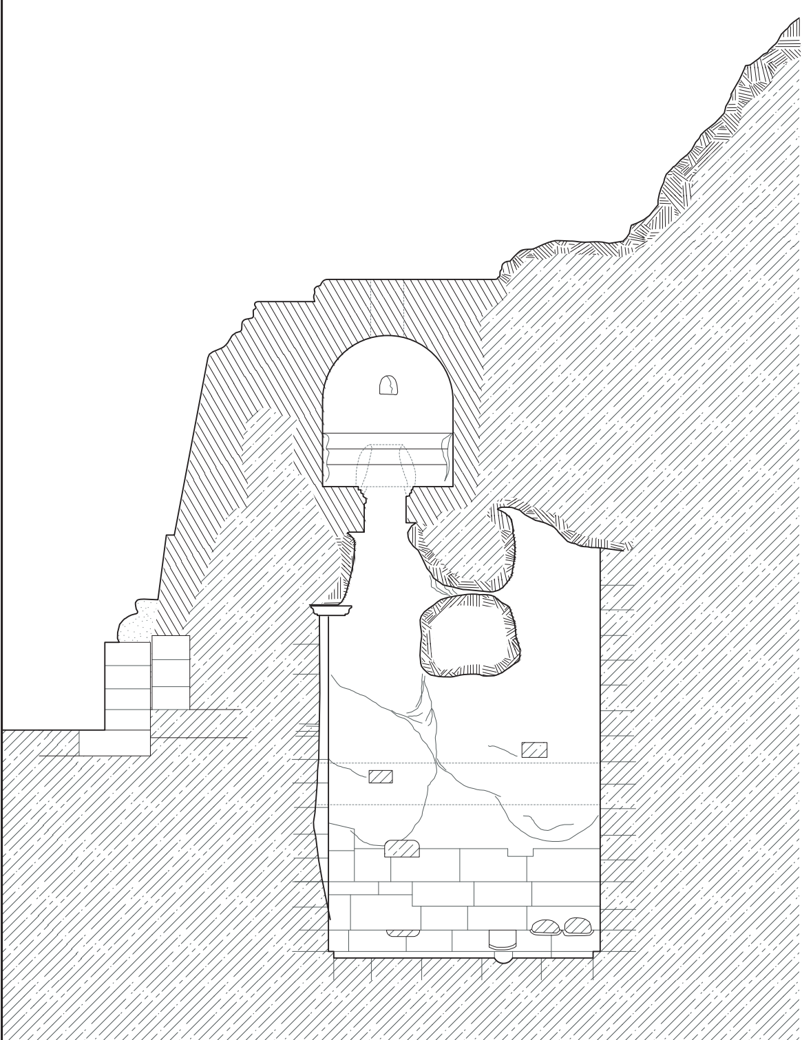
1 Fonte Klepsydra 470 - 460 a.C. pianta superiore e sezione
