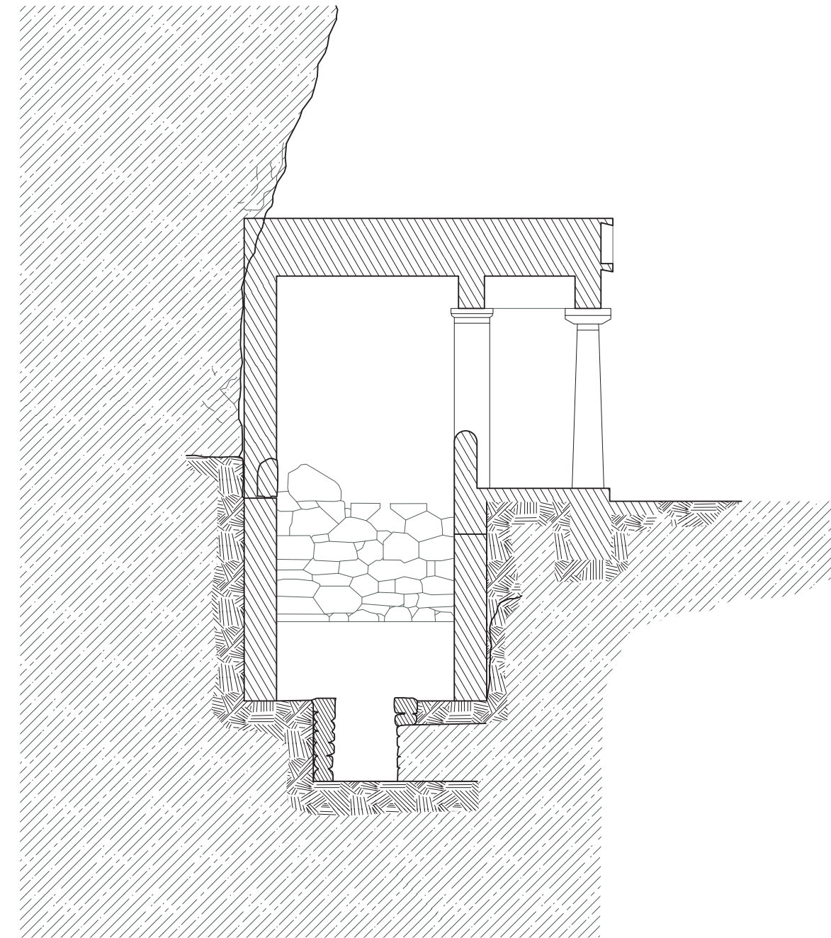
6 Krene arcaica VI secolo a.C. pianta e sezione
