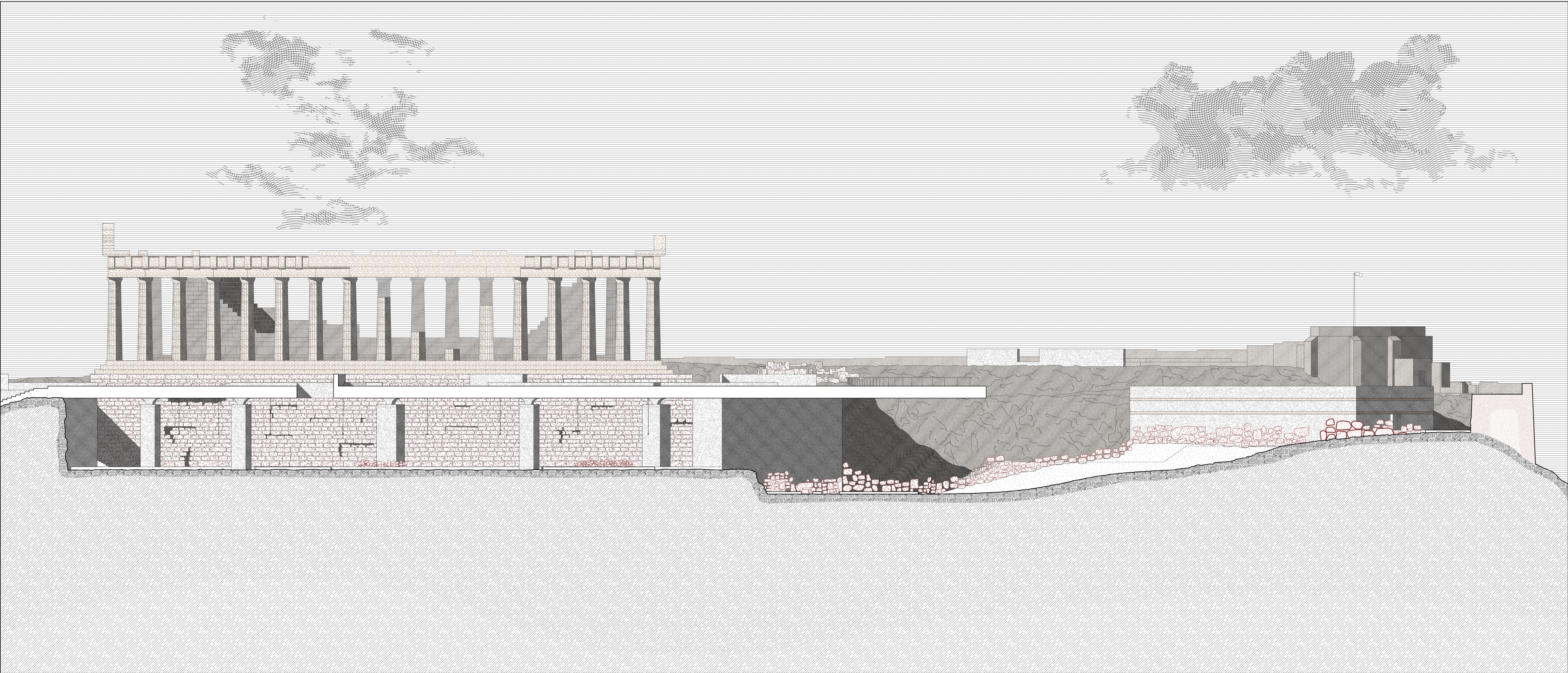
Acropoli di Atene Sezione Colmata Persiana 1:200
