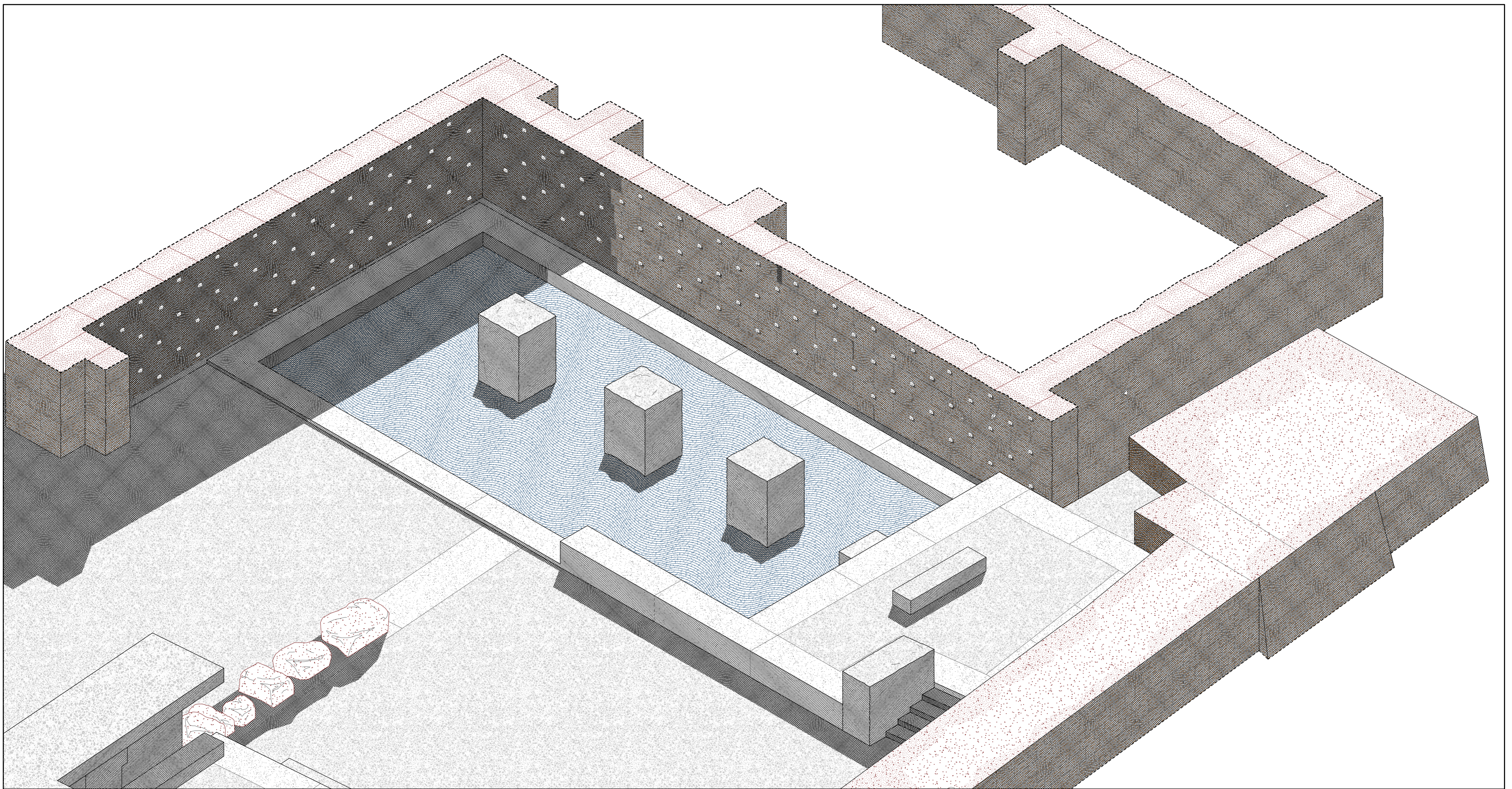
Acropoli di Atene Dettaglio di progetto - Ex cisterna 1:15 - 1:75
