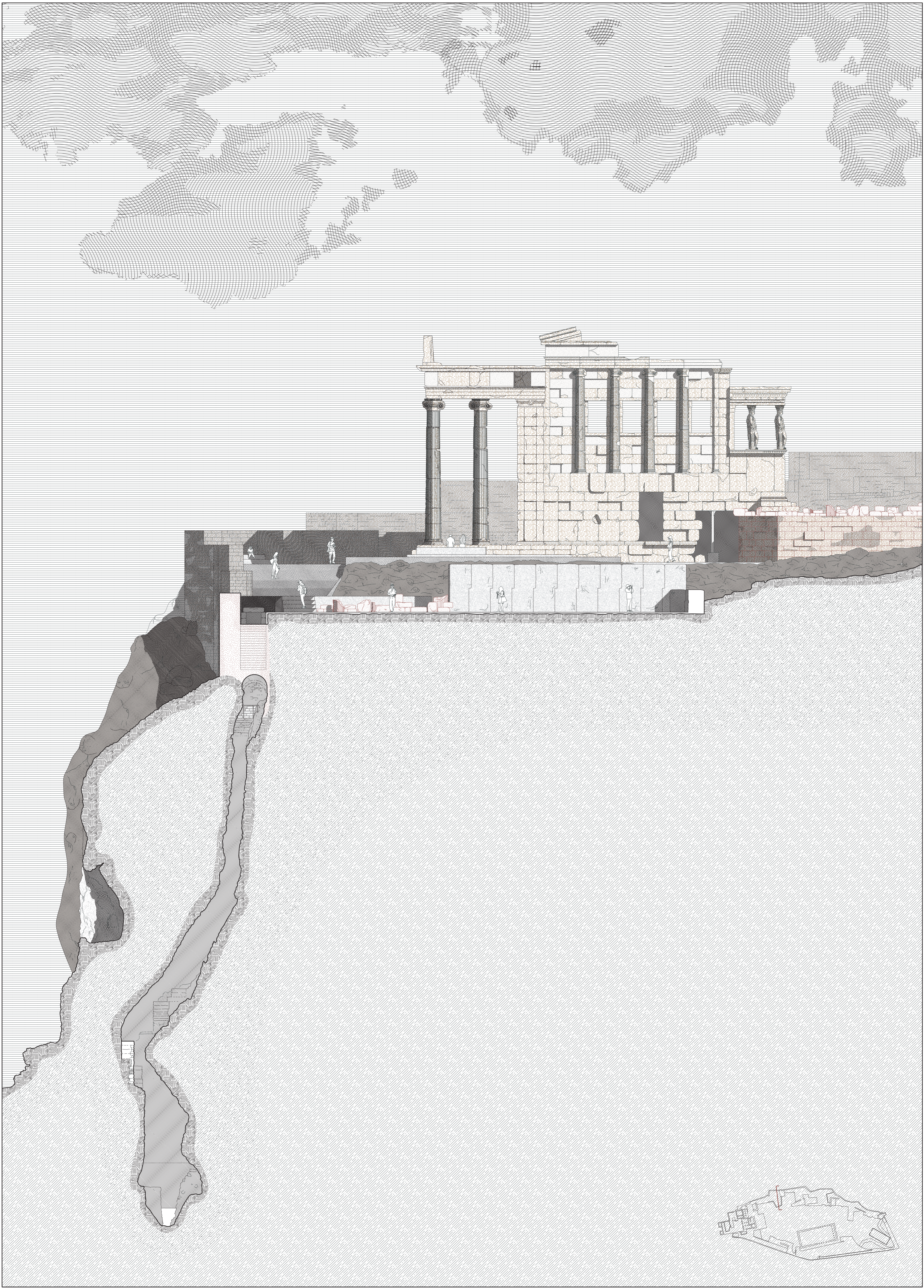
Acropoli di Atene Sezione Casa delle Arrefore 1:100
