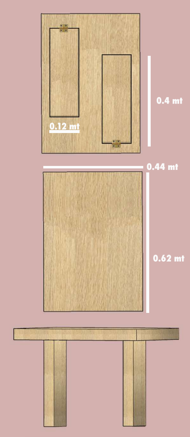
dettaglio sgabello estraibile
