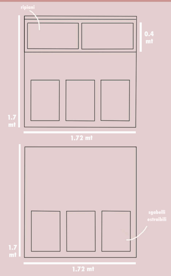
prospetti longitudinali
