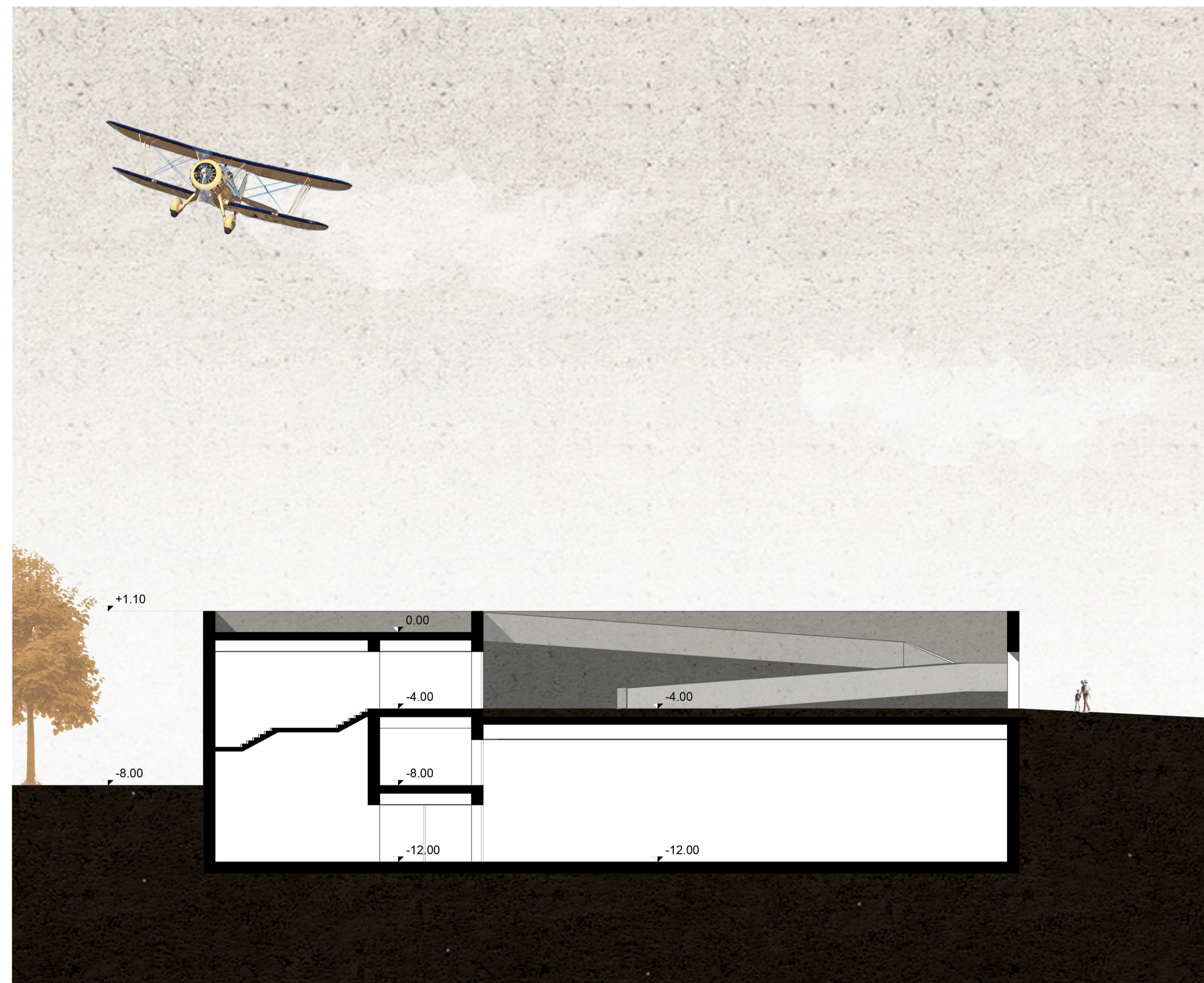
SEZIONE E-E'
