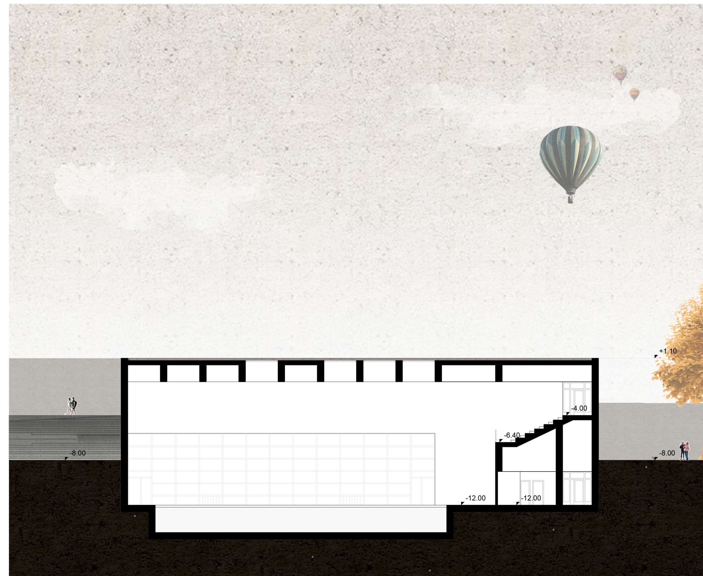
SEZIONE F-F'
