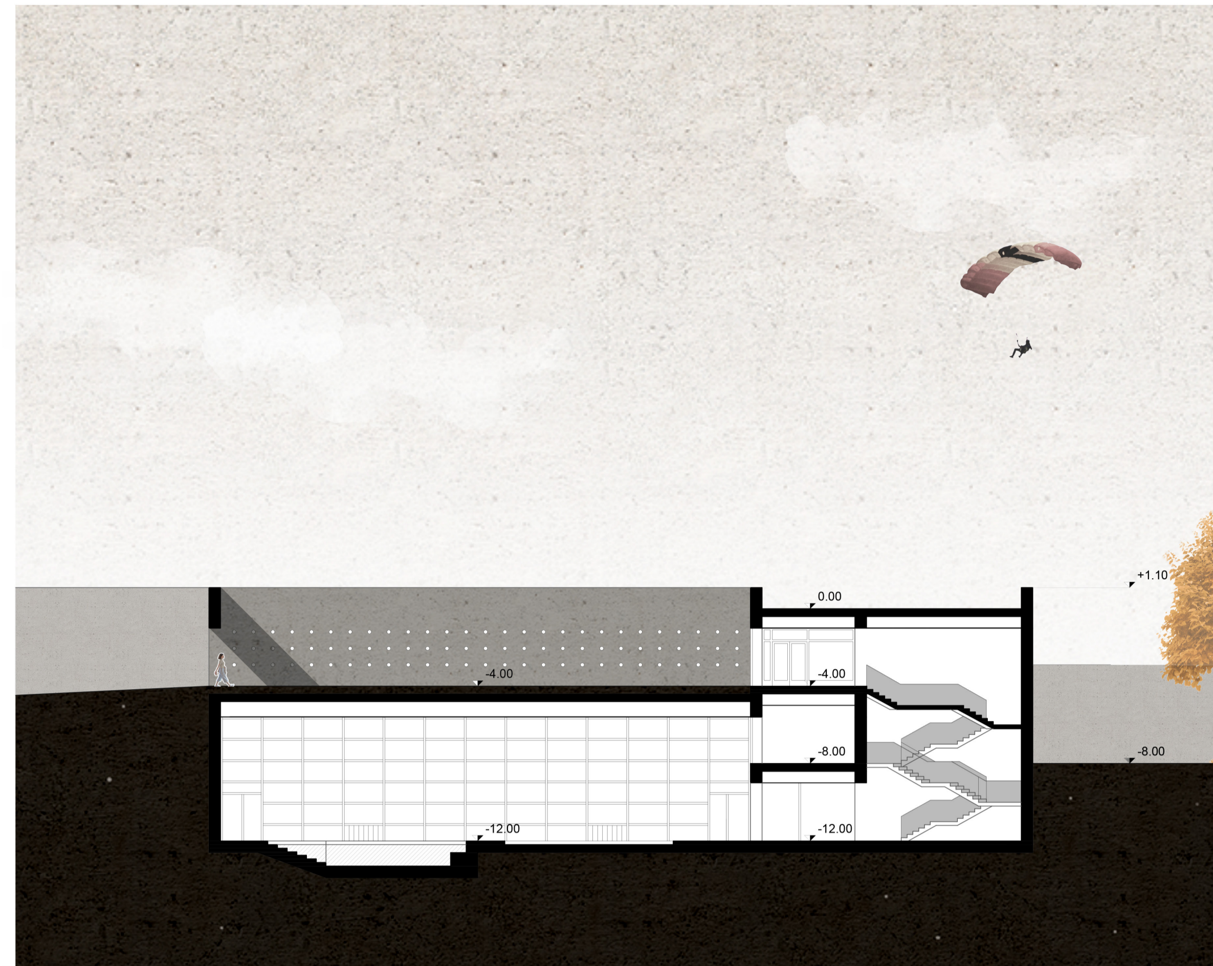
SEZIONE D-D'
