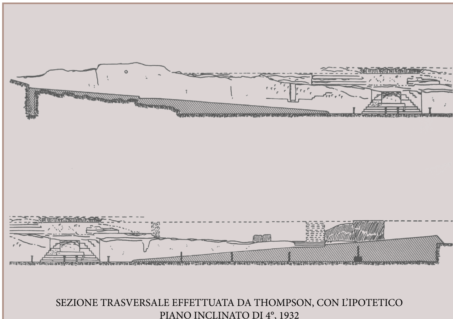
SEZIONE TRASVERSALE EFFETTUATA DA THOMPSON, CON L'IPOTETICO PIANO INCLINATO DI 4°, 1932
