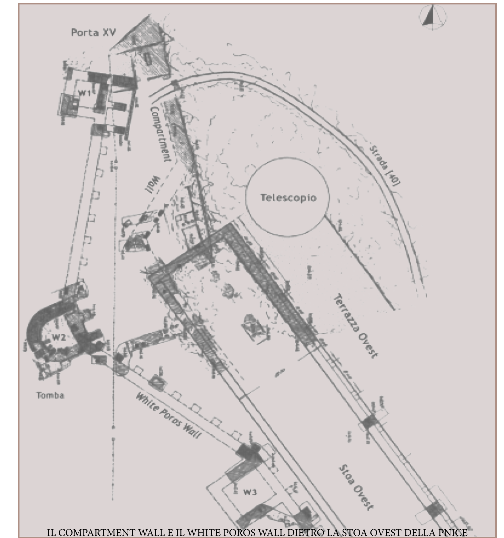
IL COMPARTMENT WALL E IL WHITE POROS WALL DIETRO LA STOA OVEST DELLA PNICE
