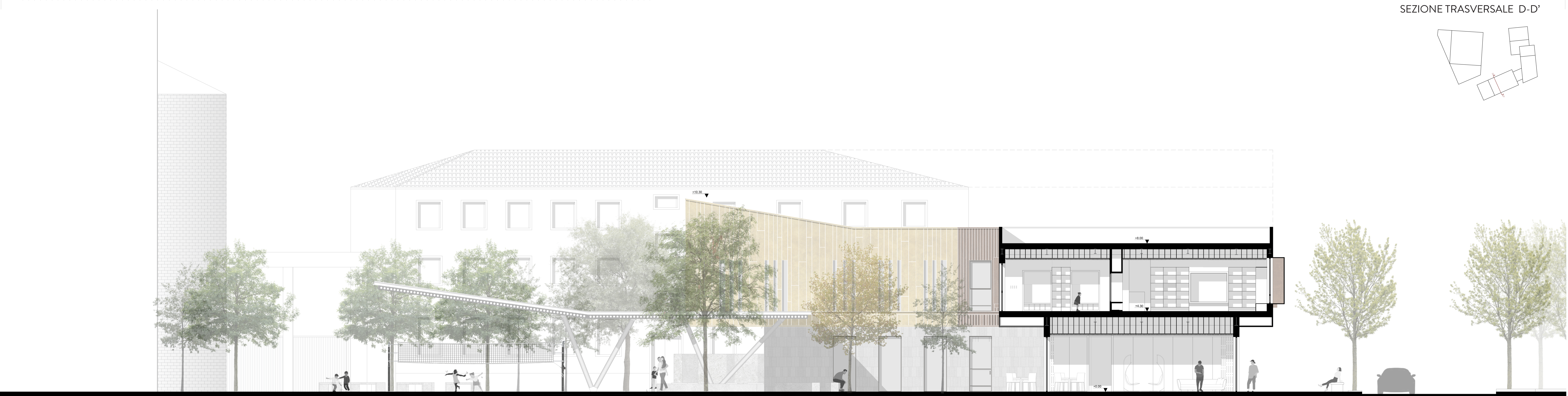
SEZIONE TRASVERSALE D-D'
