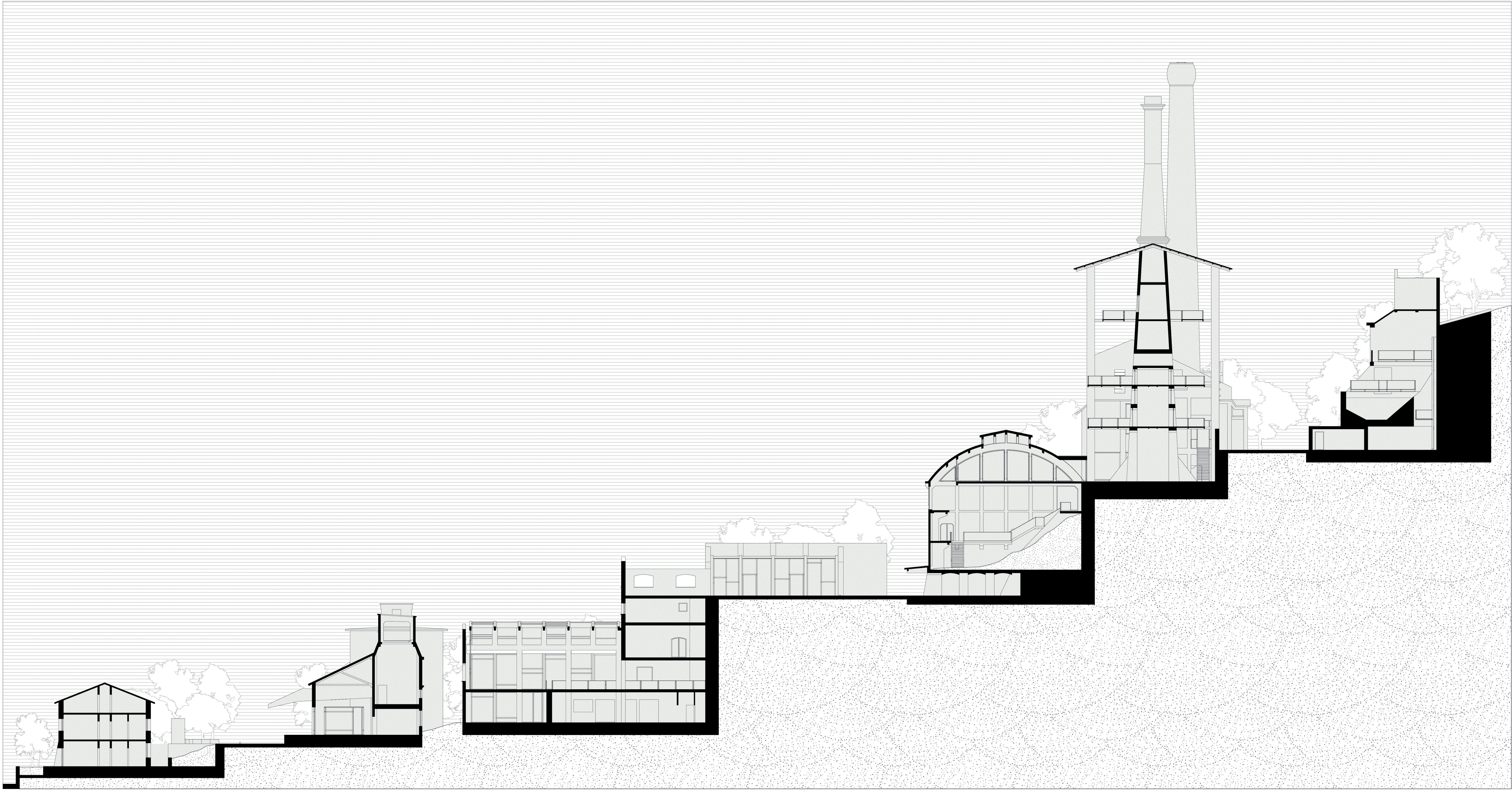
Sezione Ambientale Stato di Progetto 1:300
