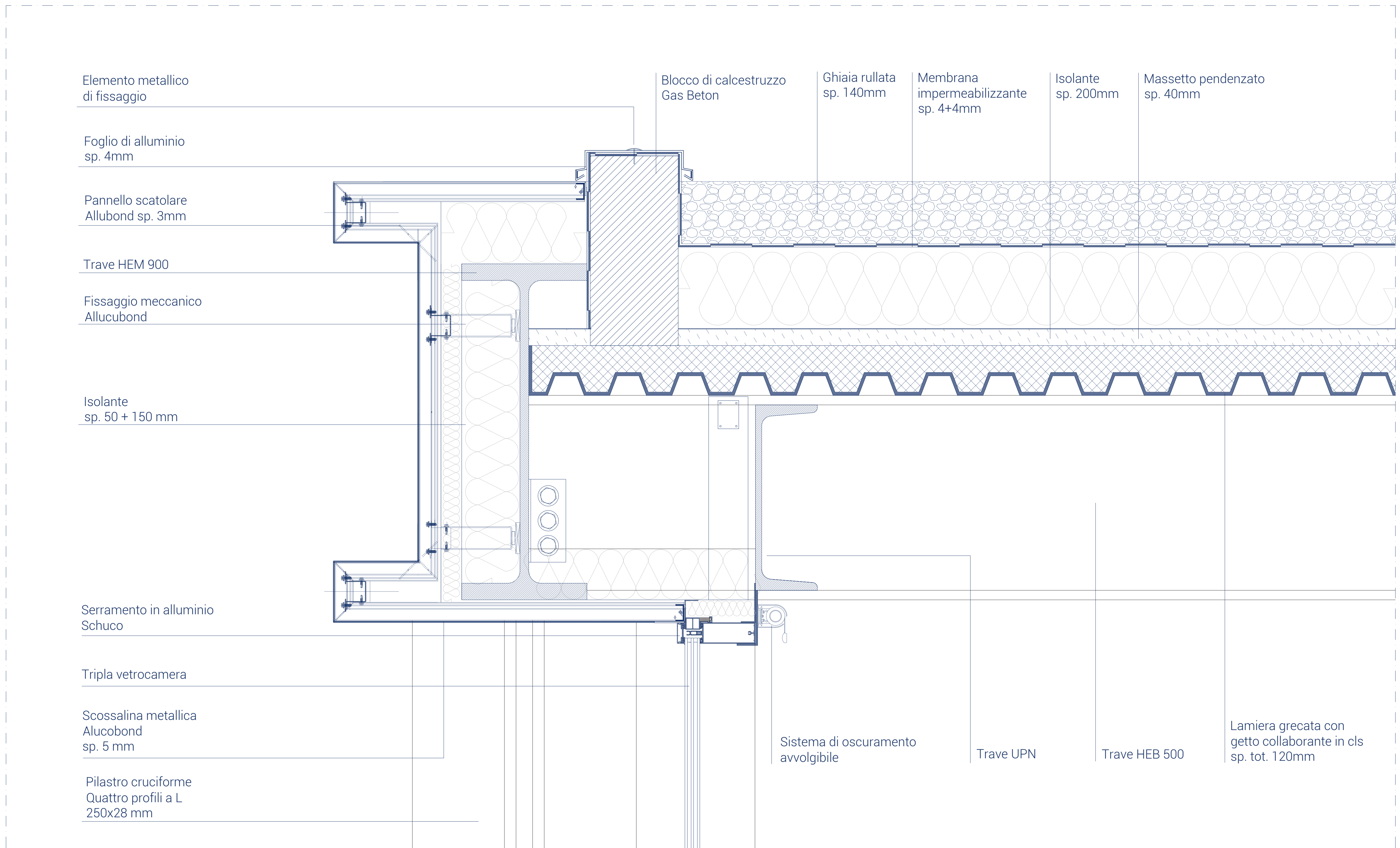
Chiusura orizzontale tipica su vetrata continua
