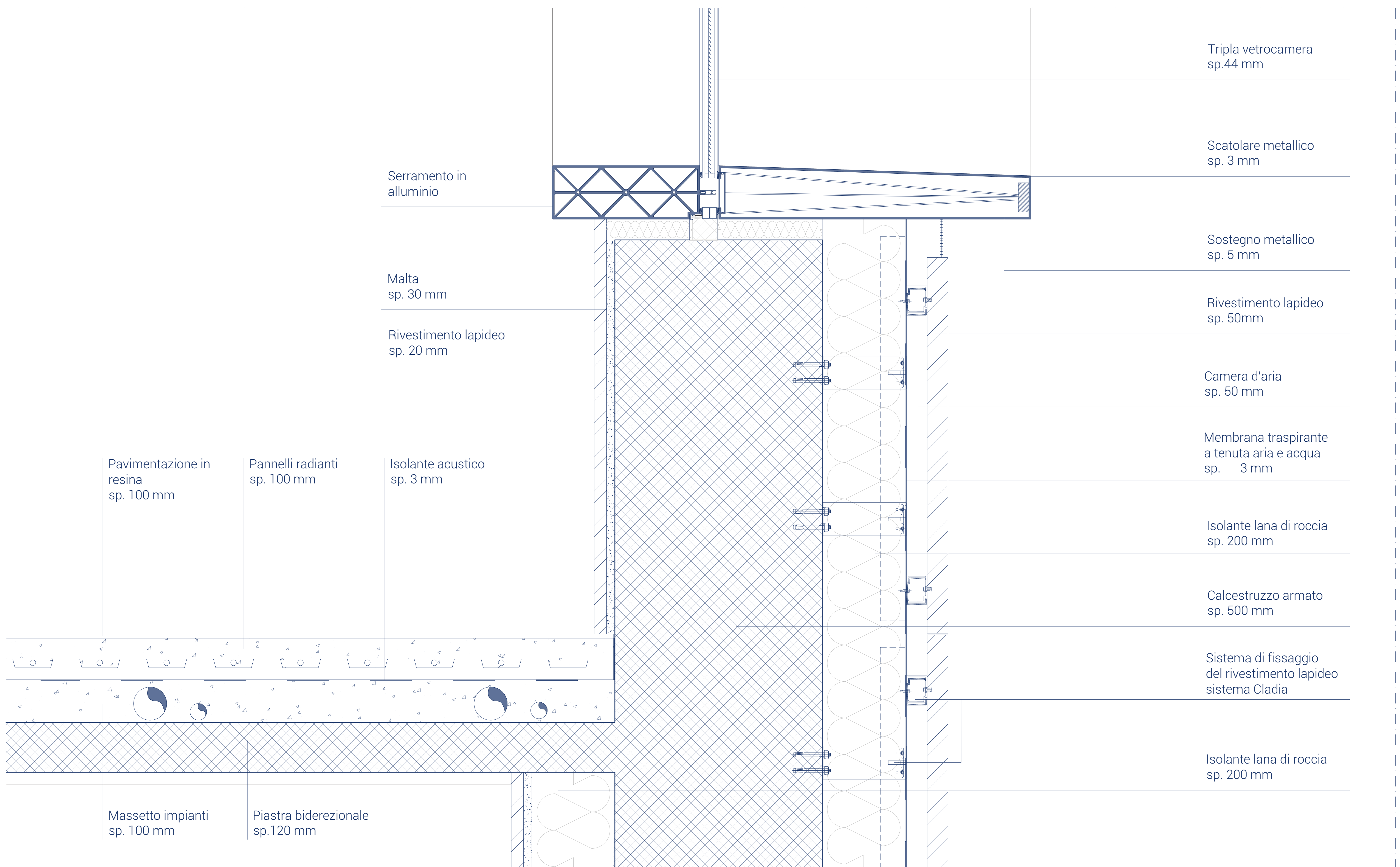
Sezione verticale tipica finestra
