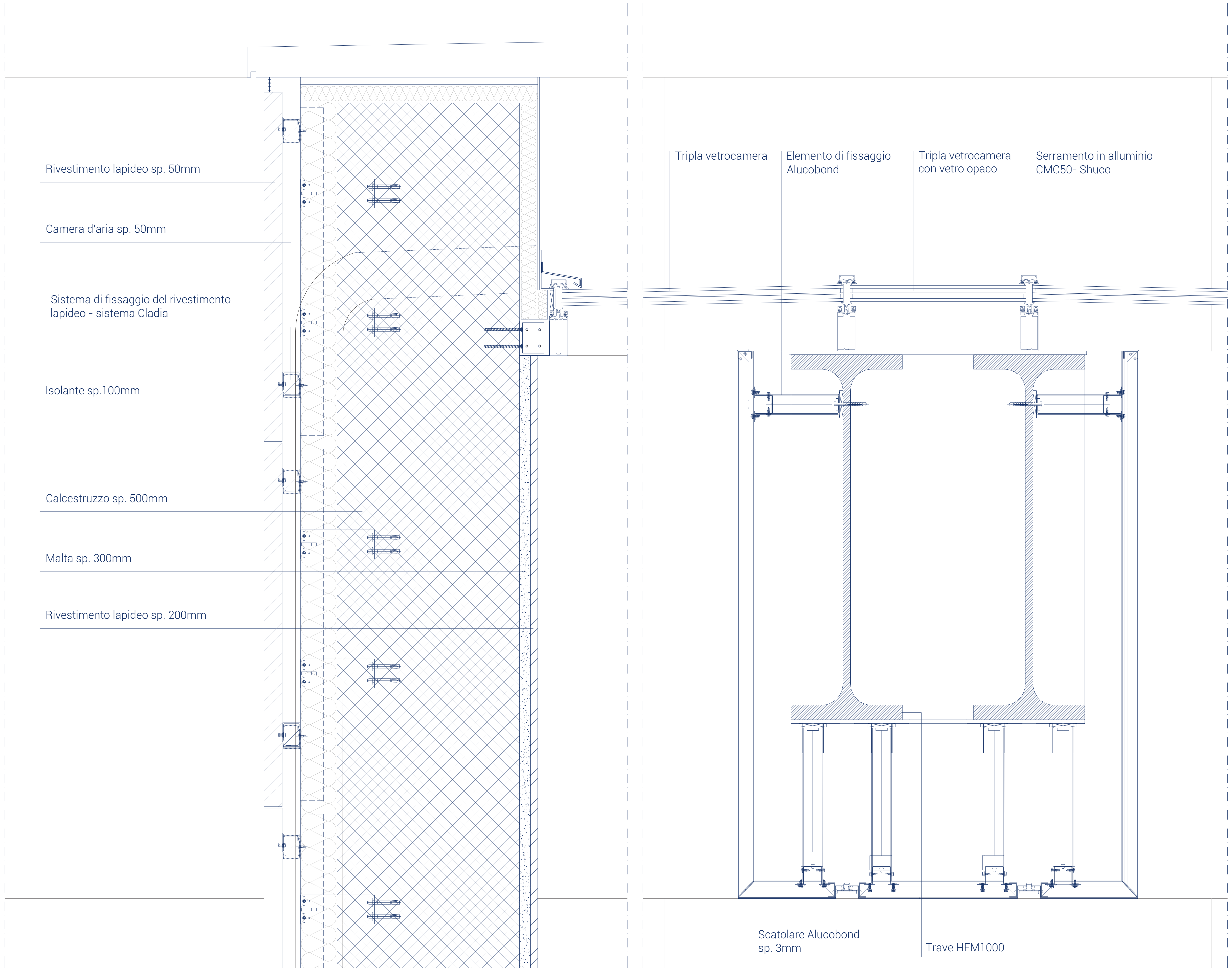
Cassettonato sala centrale
