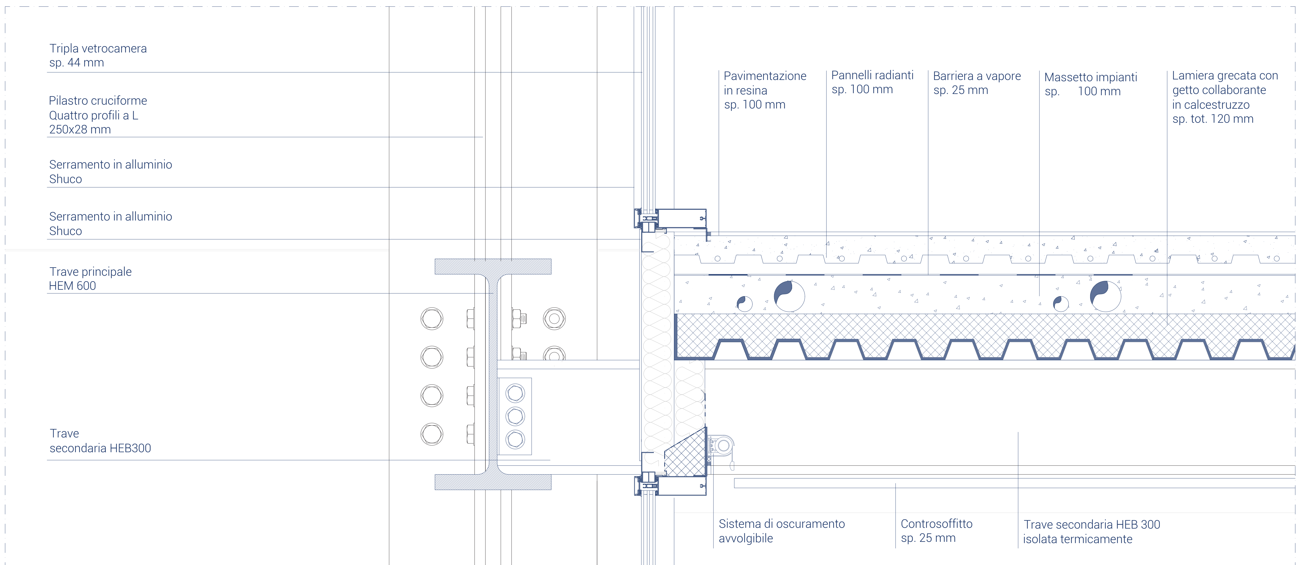
Chiusura orizzontale di interpiano mostre temporanee-restauro
