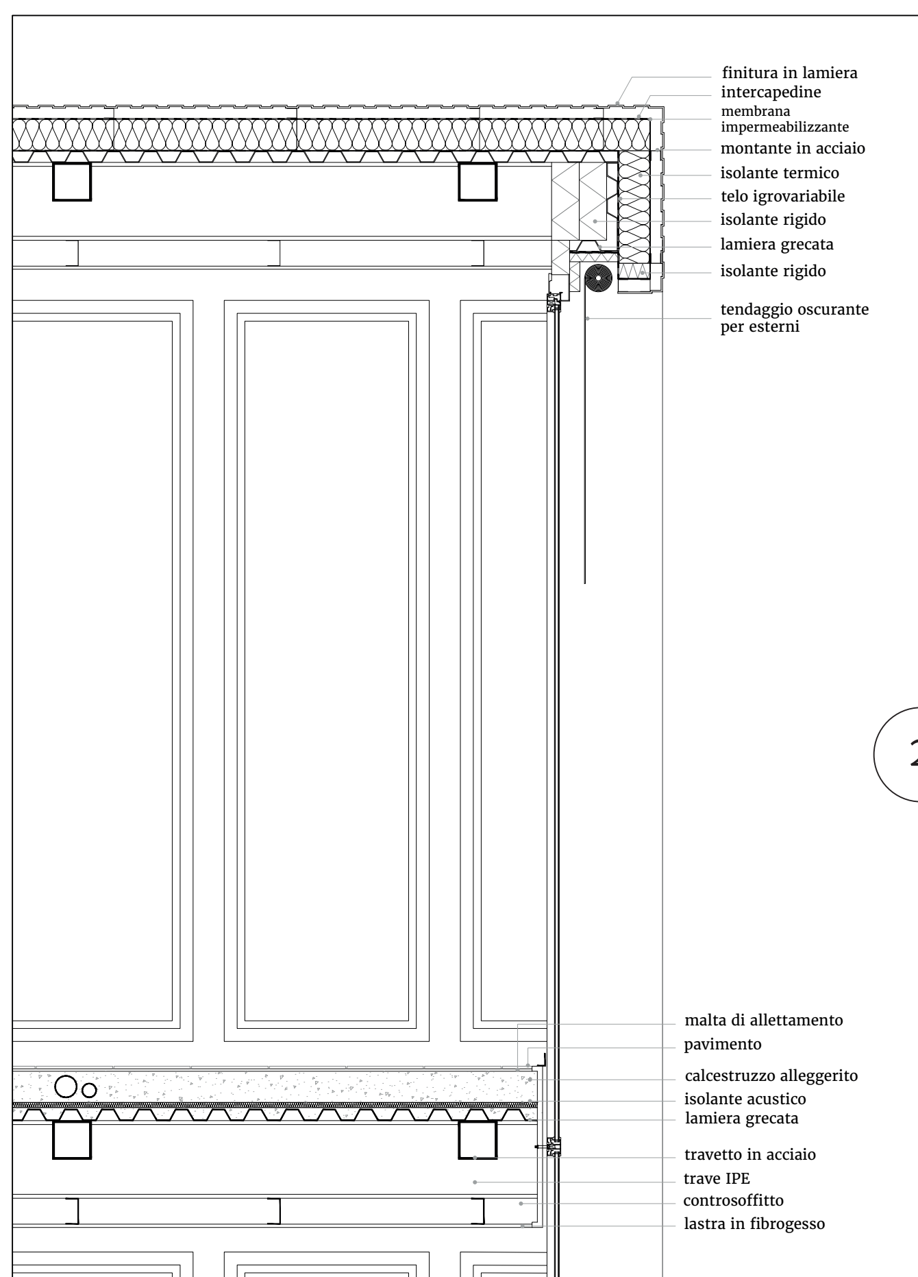
DETTAGLIO COSTRUTTIVO 1:20 - sezione - facciata continua fronte Sud
