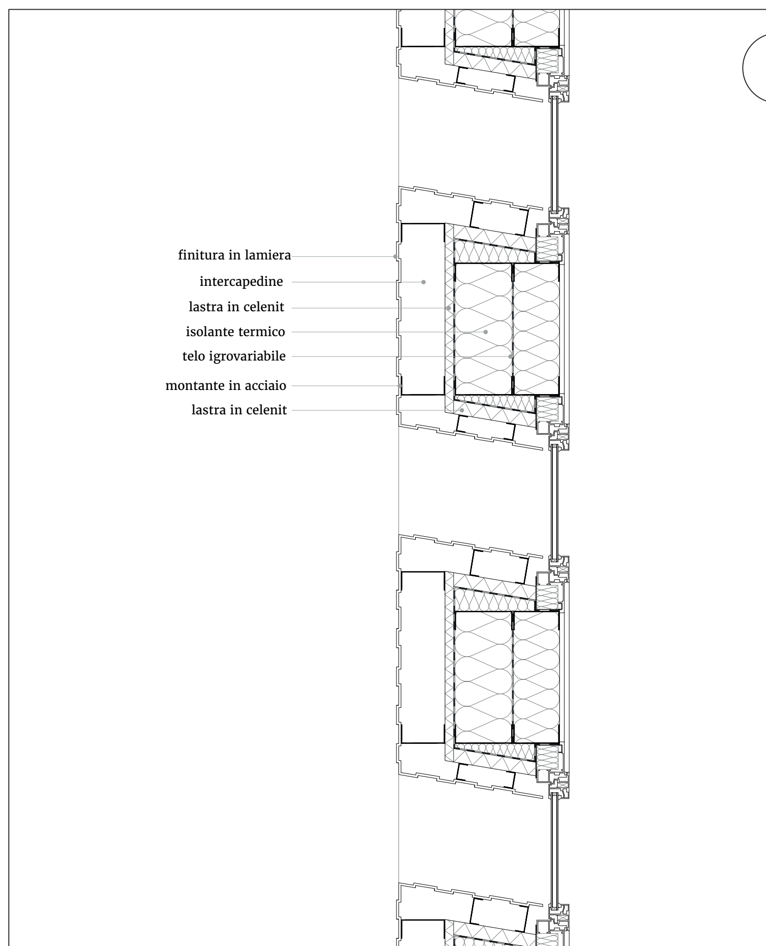
DETTAGLIO COSTRUTTIVO 1:10 - planimetria - fronte Ovest
