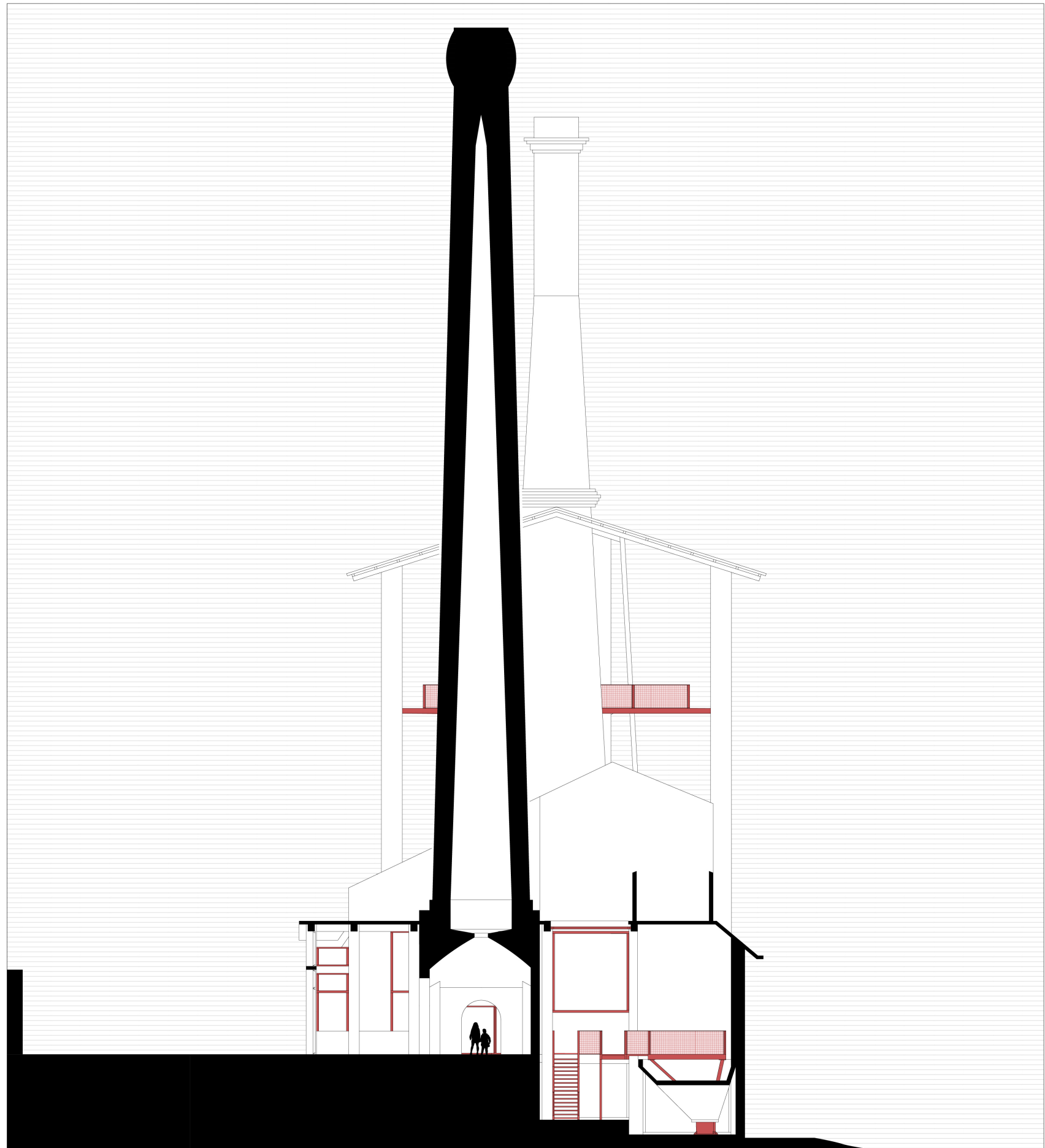
Sezione B-B'
