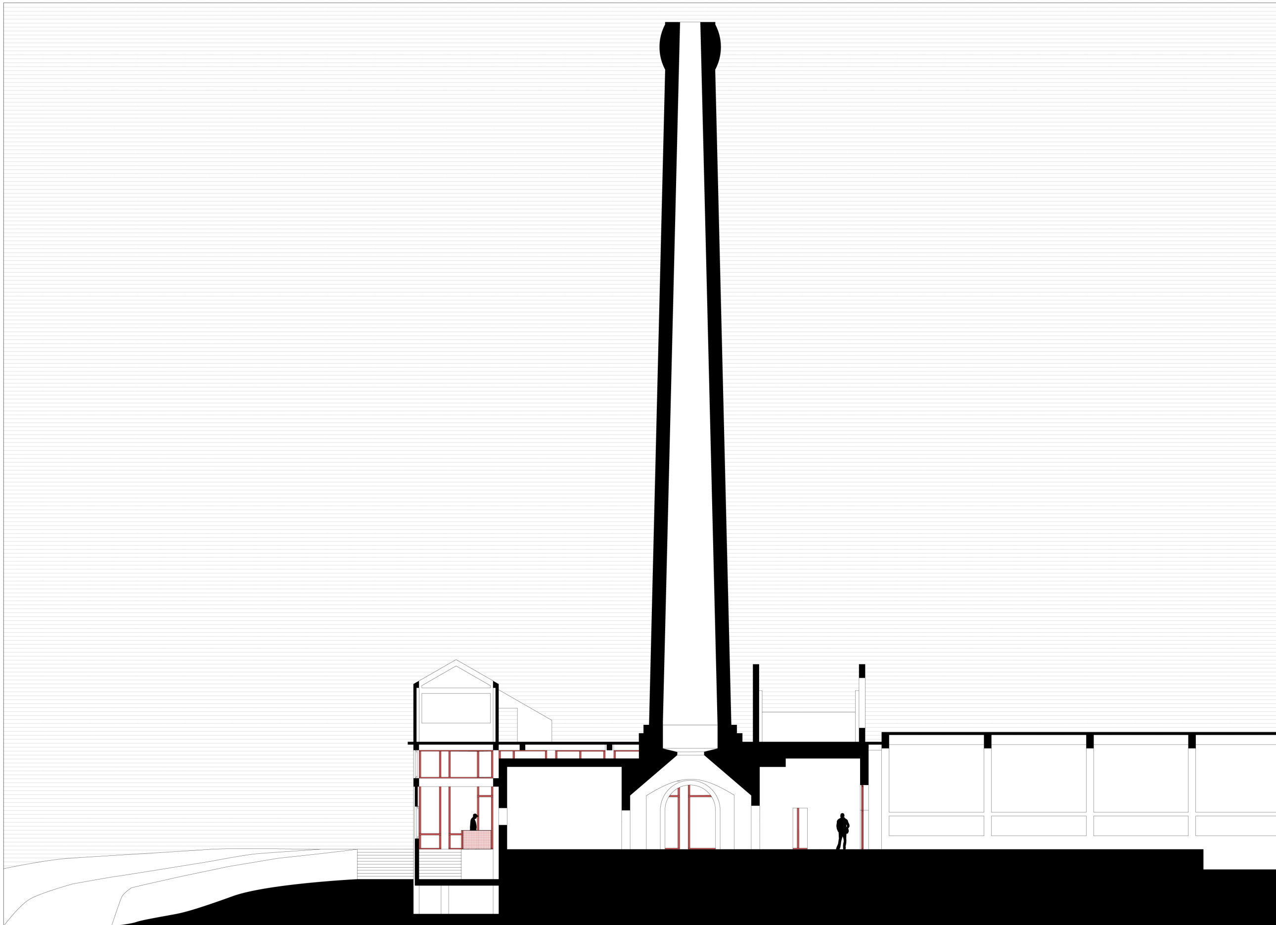
Sezione A-A'
