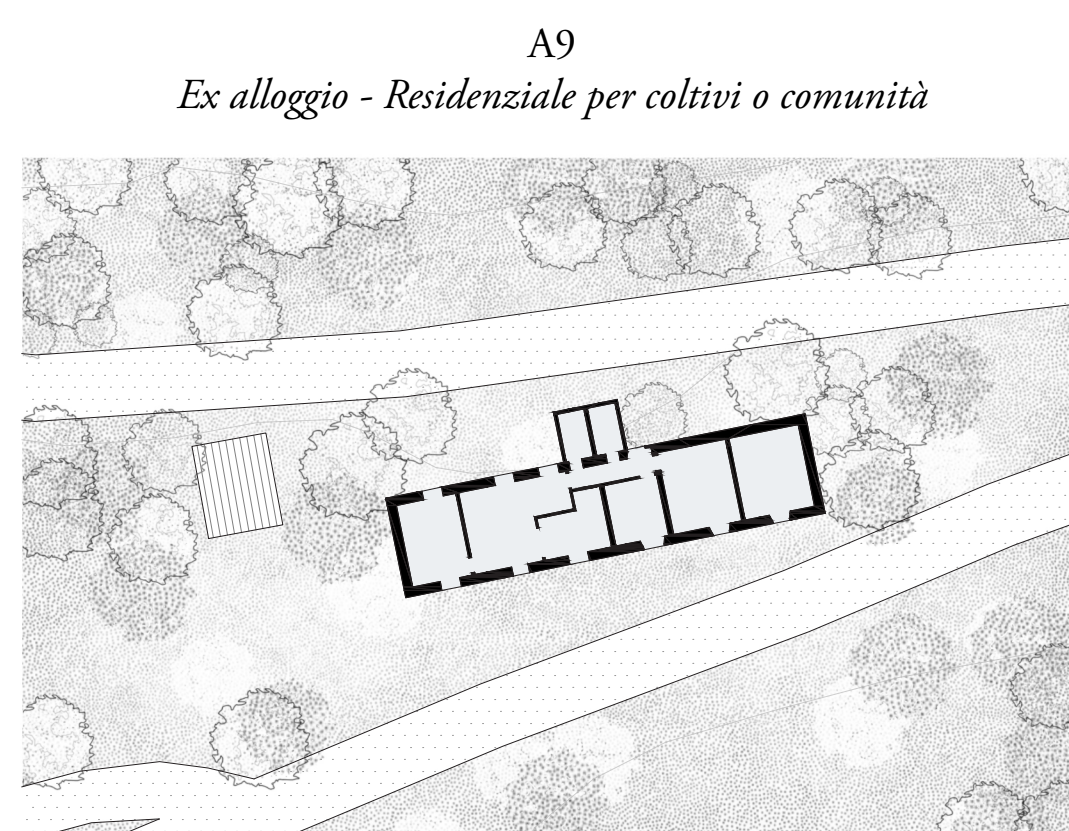
EDIFICI DA RICONVERTIRE PER RIATTIVAZIONE AGRICOLA Collegamenti e localizzazione rispetto ai terreni coltivati Scala 1:500
