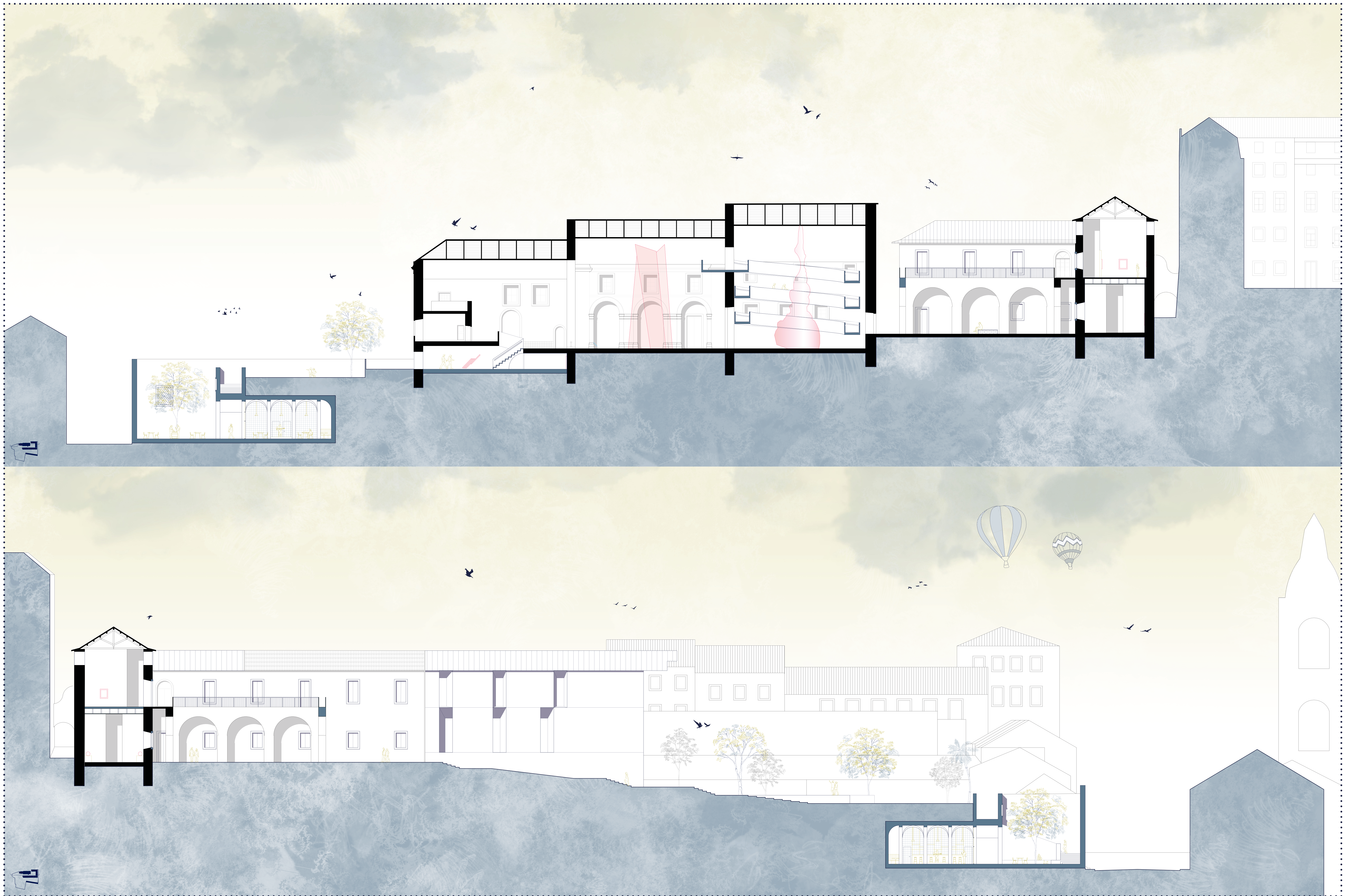
Sezioni longitudinali di progetto 1:200
