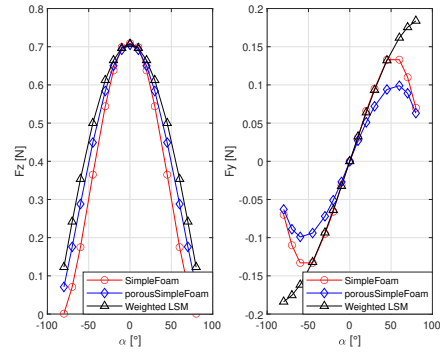
(d) Woven Wire: Weighted LSM on F_z and F_y
