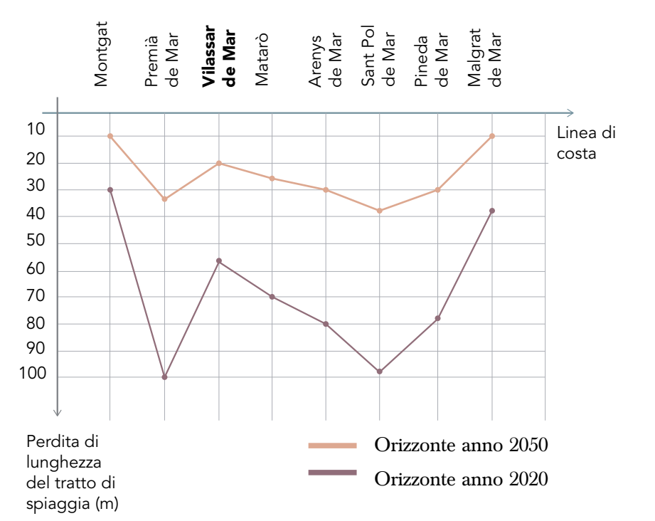
(2) Grafico dell'andamento dell'erosione nel Basso Maresme (Dati del Rapporto Tecnico del Ministero dell'agricoltura, dell'alimentazione e dell'ambiente)
