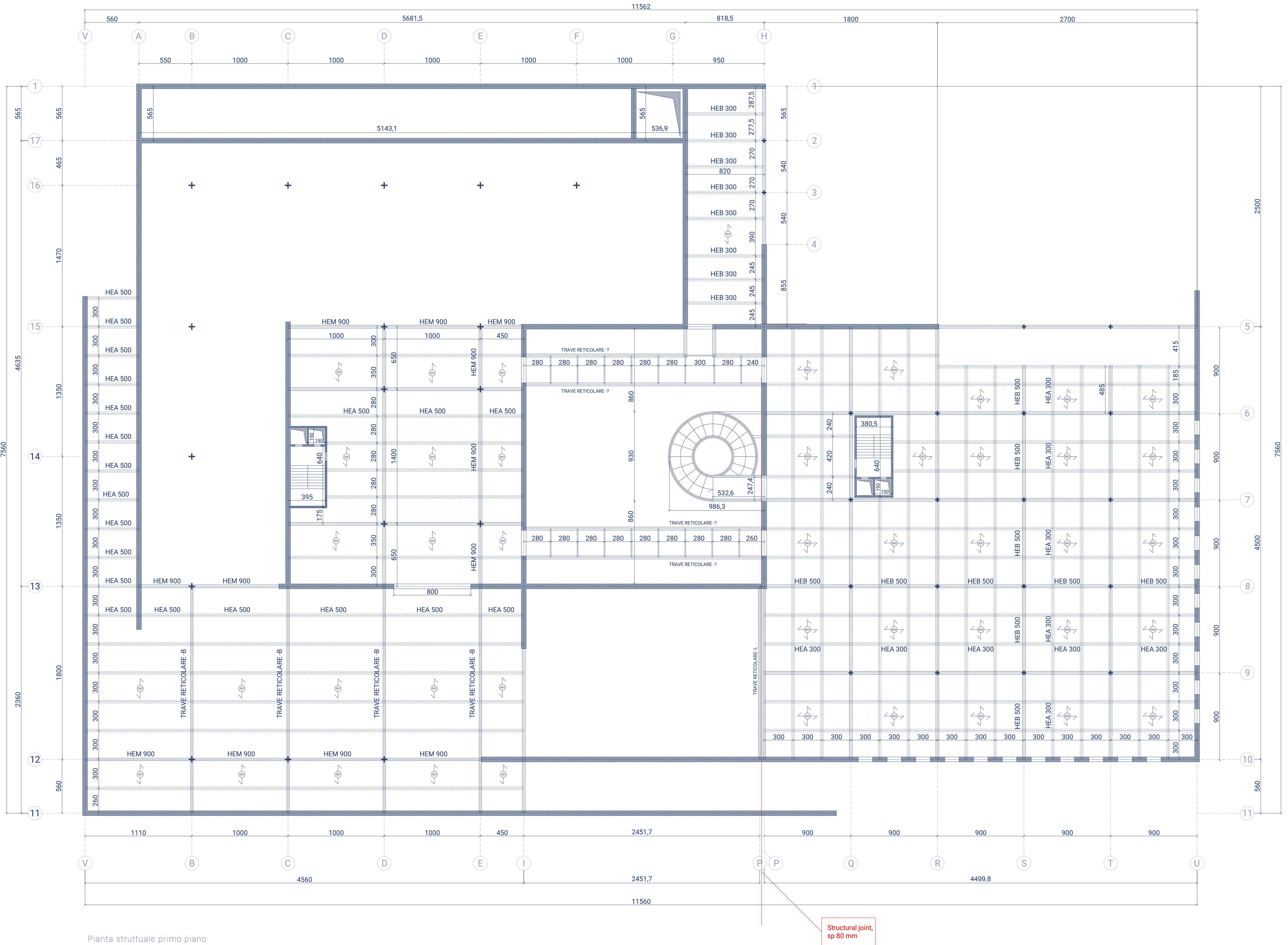
Pianta strutturale primo piano
