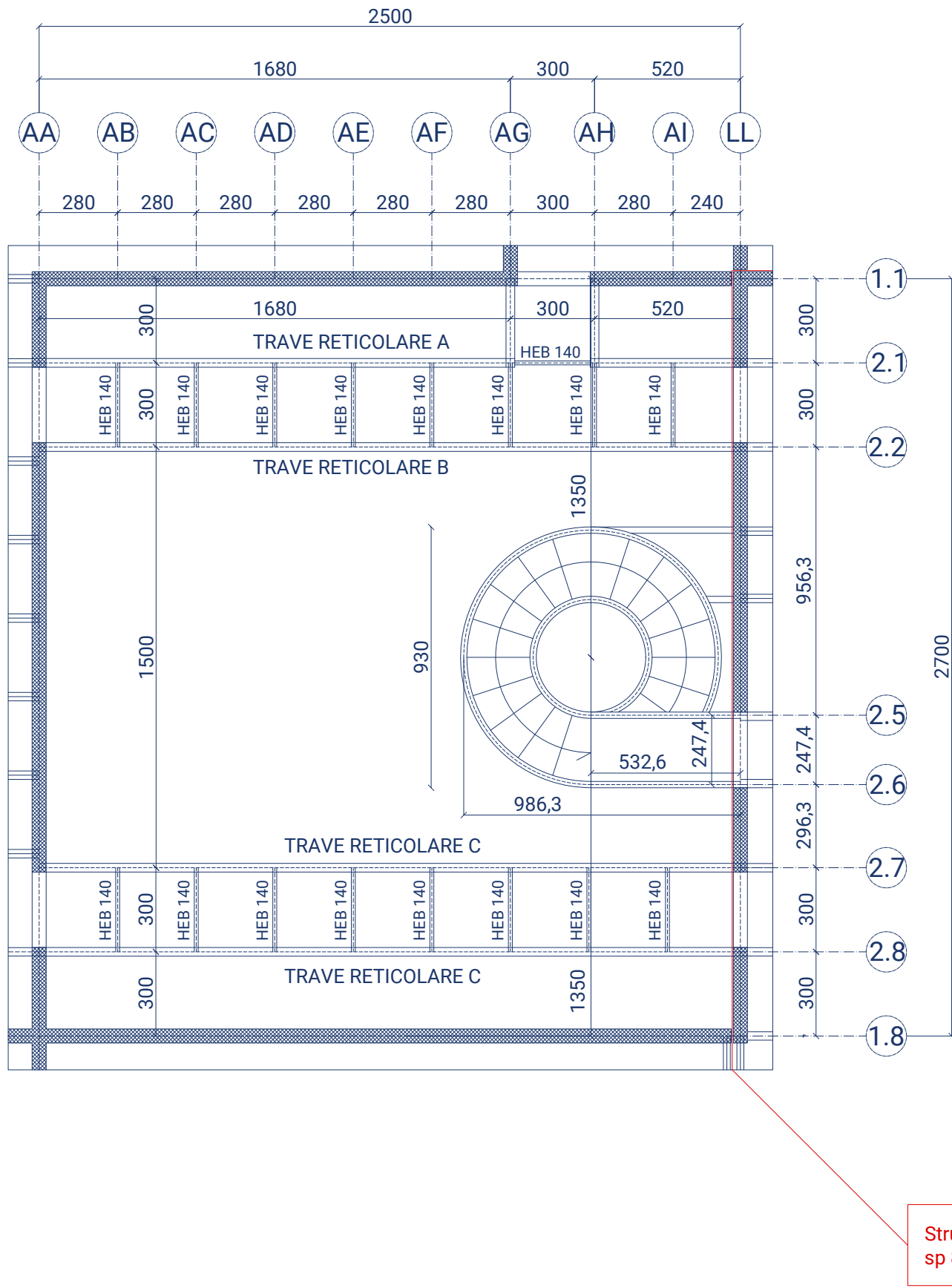
Pianta strutturale primo piano - sala centrale
