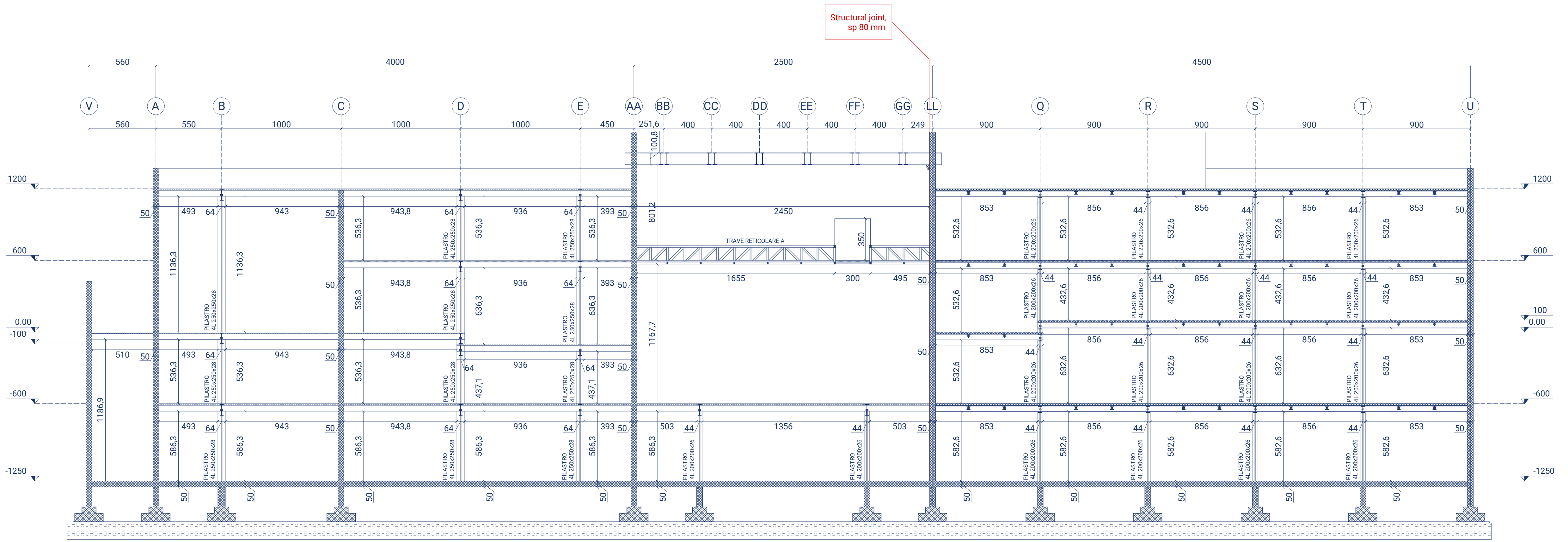
Sezione longitudinale strutturale
