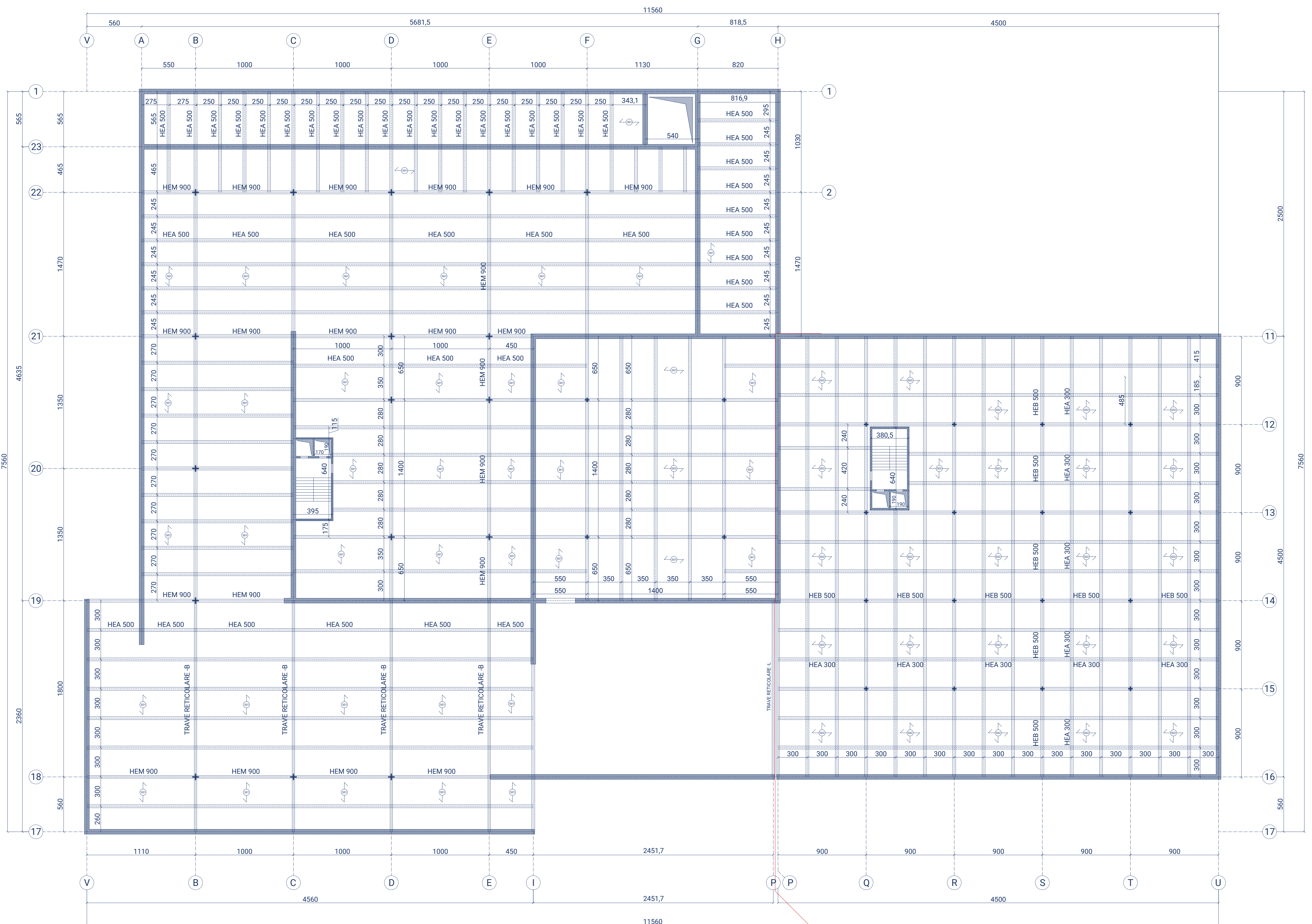
Pianta strutturale primo piano interrato
