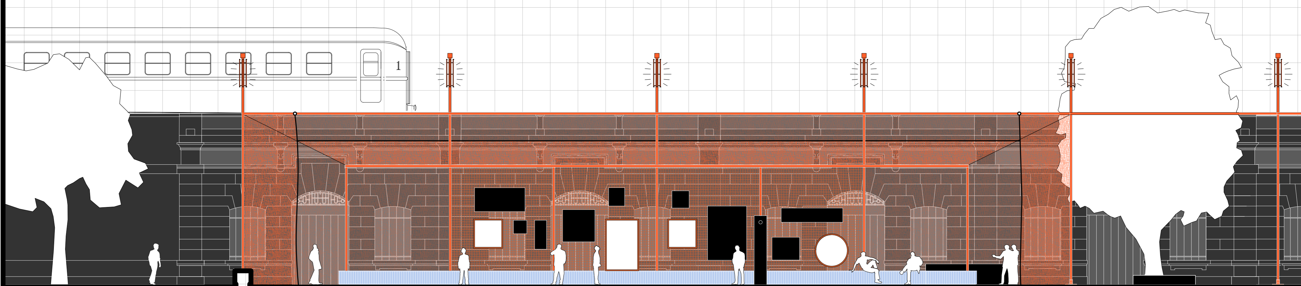
Sezione longitudinale 1:100
