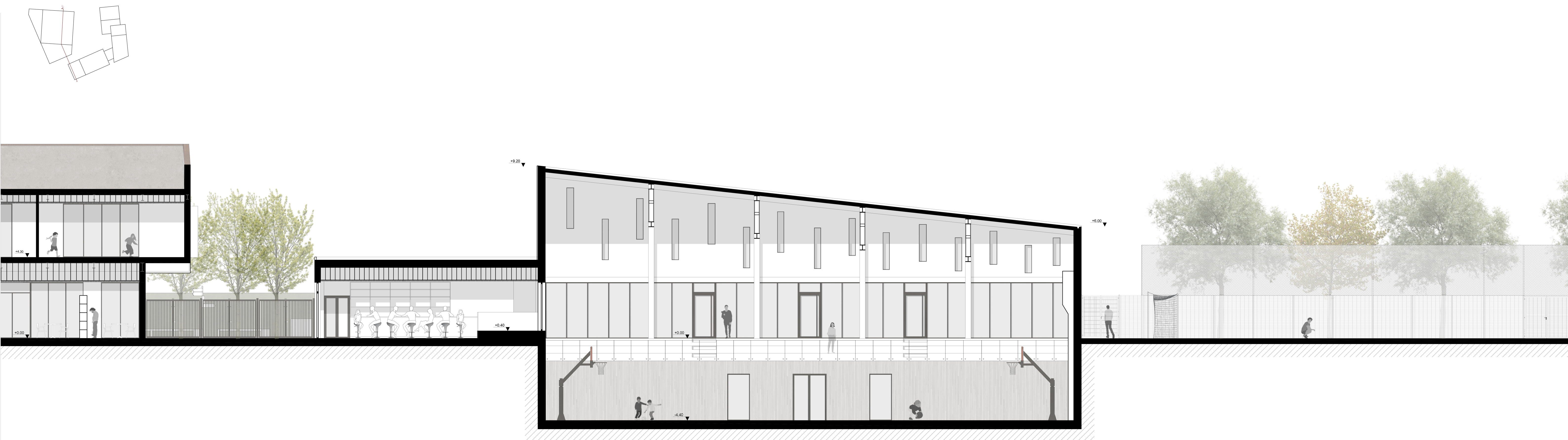
SEZIONE LONGITUDINALE PALESTRA G-G'
